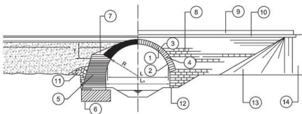
Slika 2.20. Poprečni presjek svođenog propusta (elementi: 1 – svod; 2 – intrados; 3 – ekstrados; 4 – peta svoda; 5 – upornjak; 6 – temelj; 7 – nazidak; 8 – čeonu zid; 9 – ograda; 10 – vijenac; 11 – kameni nabačaj; 12 – profil kanala; 13 – čunj; 14 – prilaz mostu; L – raspon svoda; L_0 – otvor propusta; r – radijus zakrivljenosti svoda; f – strelica svoda) (Izvor: Cerić i sur., 2022.)
