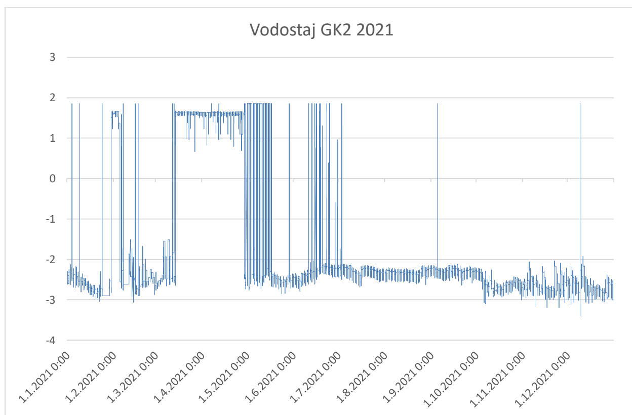
Graf 3.3. Razine vodostaja na postaji monitoringa GK 2 tijekom 2021. godine
