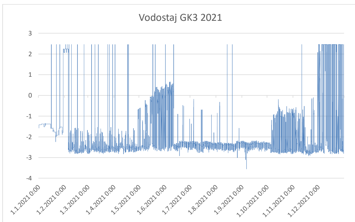
Graf 3.5. Razine vodostaja na postaji monitoringa GK 3 tijekom 2021. godine
