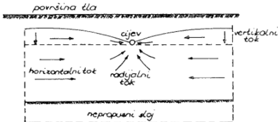
Slika 2.10. Vertikalni, horizontalni i radijali tok vode (izvor: Tomić 1987.)
