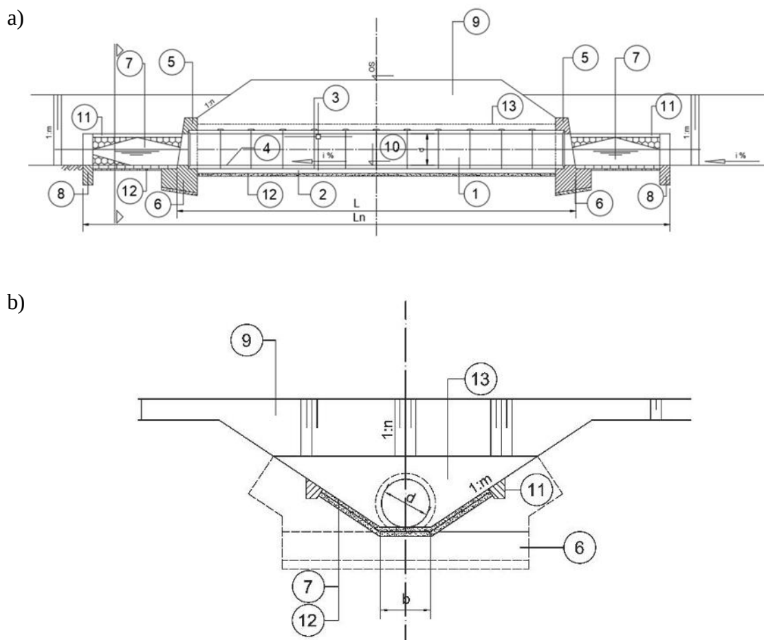
Slika 2.19. Presjeci cijevnog propusta: a) uzdužni presjek, b) poprečni presjek (1 – cijev; 2 – podloga; 3 – spoj cijevnih elemenata; 4 – niveleta, dno propusta; 5 – čeoní zid; 6 – temelj čeonog zida; 7 – obloga kanala; 8 – prag; 9 – trup prometnice; 10 – kota dna propusta; 11 – pasica; 12 – posteljica; 13 – betonska ovojnica cijevnog propusta; L – duljina cijevnog propusta; Ln – duljina građevine; i – uzdužni pad nivelete; d – promjer cijevi; b – širina dna kanala) (Izvor: Cerić i sur. 2022.)
