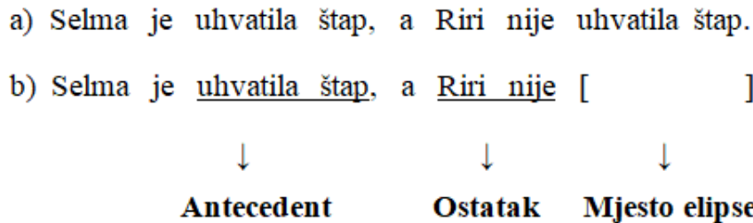
Slika 1.1. Eliptična rečenica.
