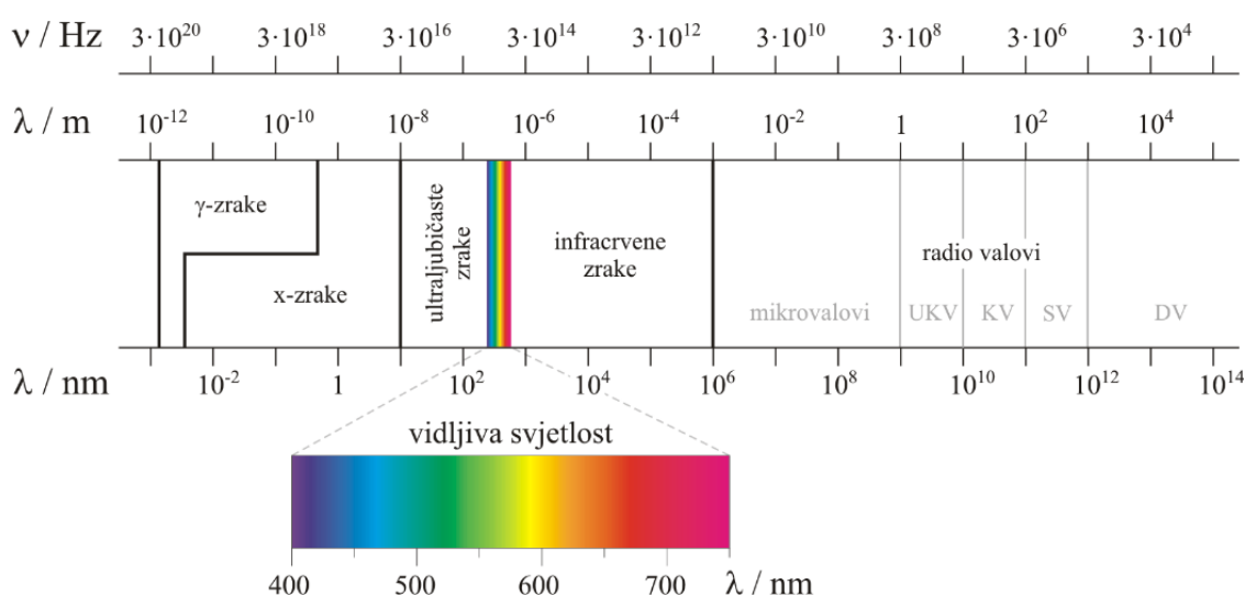
Slika 14. Elektromagnetski spektar.
