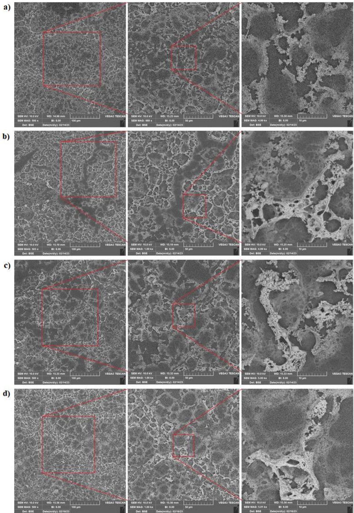
Slika 13. SEM mikrofotografije \text{LaMnO}_3 tankih filmova: a) IPL_lim3_1a, b) IPL_lim3_1b, c) IPL_lim3_2 i d) LMO_lim3_IPL snimljene pri povećanjima od 500x, 1000x i 5000x
