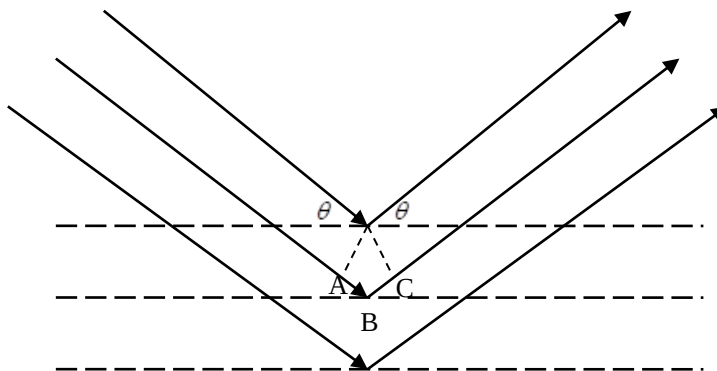
Slika 2.6. Difrakcija rendgenskih zraka na kristalu [30].
