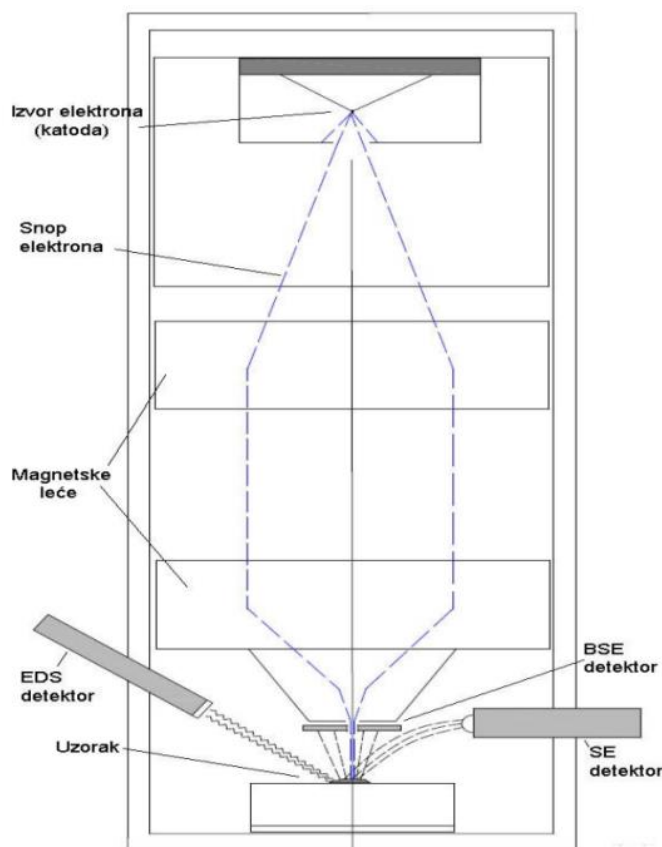
Slika 2.5. Shema SEM-a. [29]
