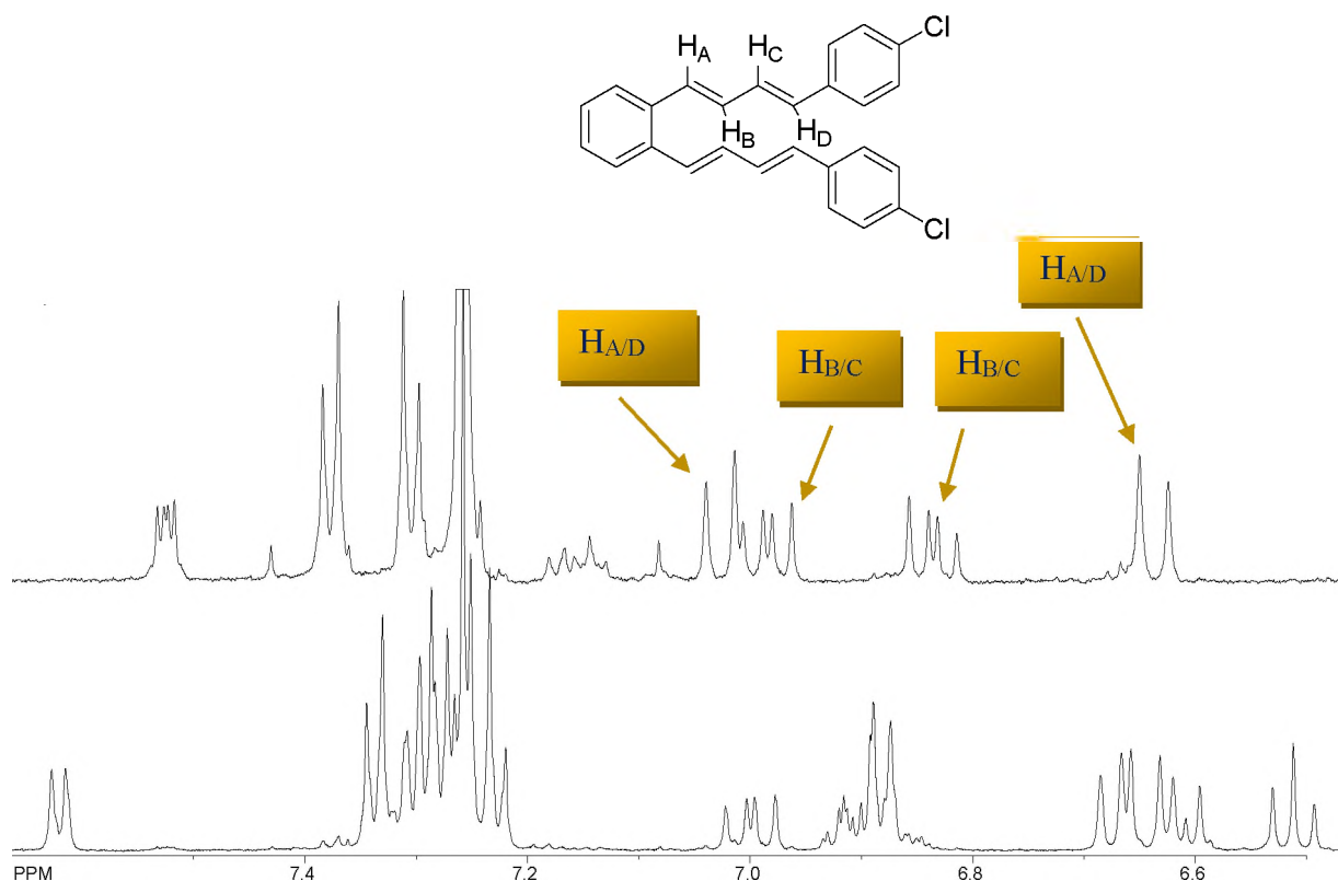
Slika 1. ^1\text{H} NMR spektri trans,trans - i cis,trans -1 izomera
