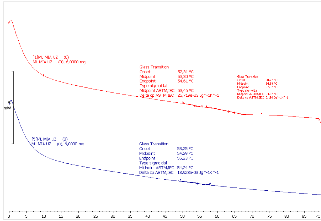
Slika 43. Termogram uzorka 10
