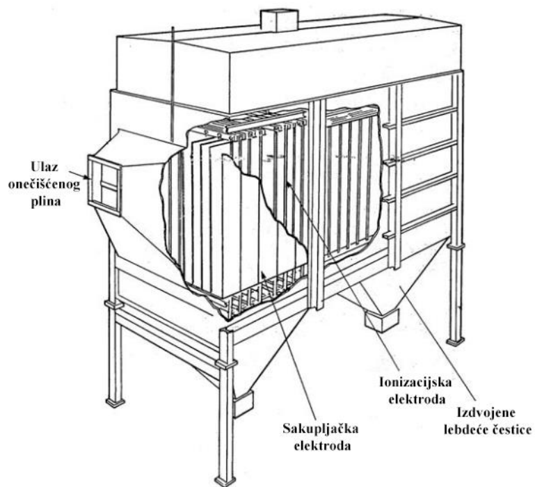
Slika 22. Elektrofiltar [59]
