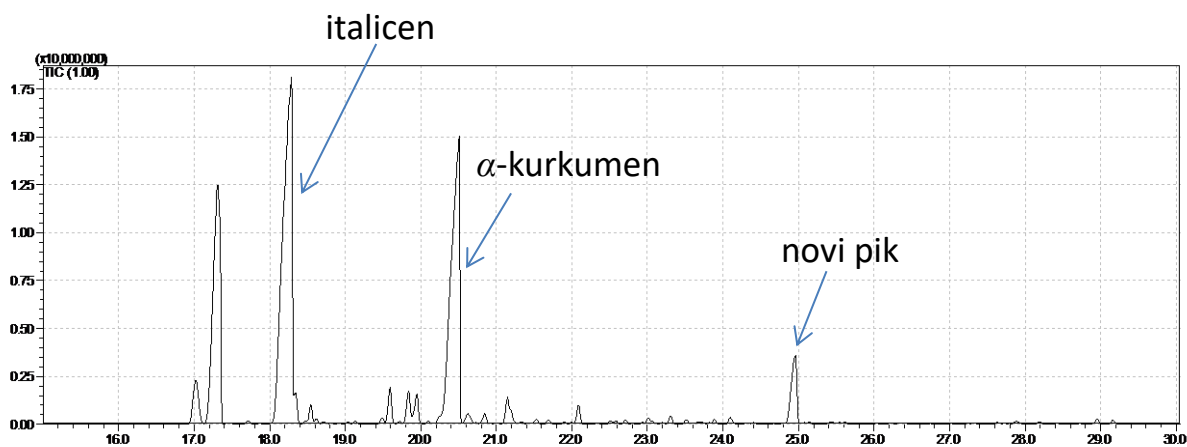
Slika 25. a) Prikaz kromatograma početne frakcije \gamma -kurukemna b) Prikaz kromatograma frakcije \gamma -kurkumena nakon osvjetljavanja od 48 h sa plinom argonom
