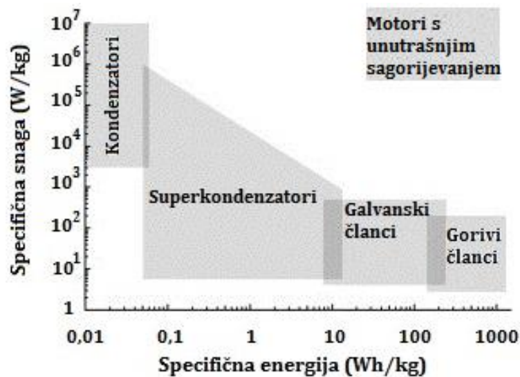
Slika 2.10 Ragoneov dijagram
