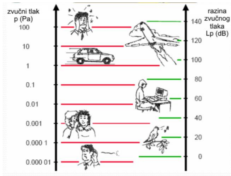
Slika 13 Usporedba zvučnog tlaka i razine zvučnog tlaka, IZVOR: [11]
