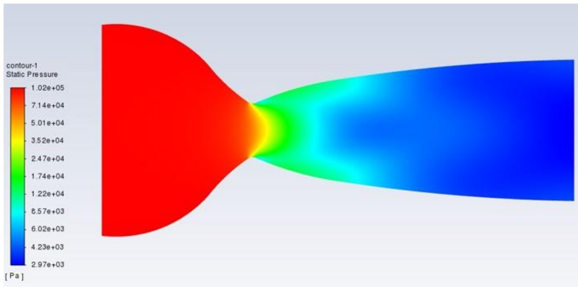
Slika 44. Distribucija statičkog tlaka pri neviskoznom strujanju, [9]
