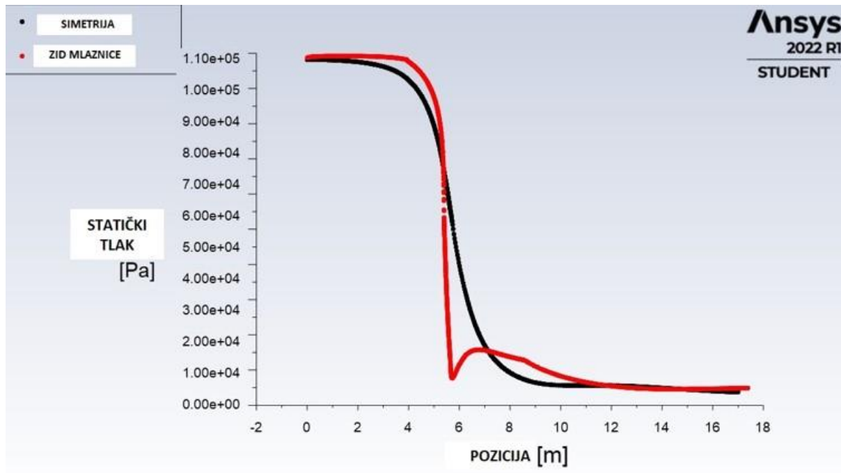
Slika 51. Grafički prikaz raspodjele tlaka na osi simetrije i zidu mlaznice, [9]
