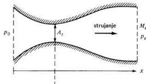
Slika 13. Konvergentno-divergentna mlaznica, [1]
