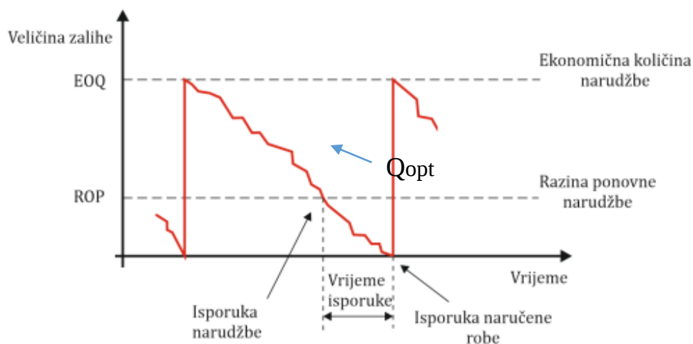
Slika 42. Interakcija razine ponovne narudžbe i vremena isporuke [11]
