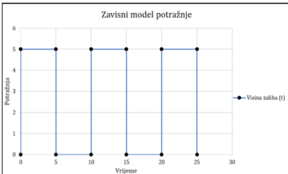
Slika 36. Zavisni model potražnje [11]
