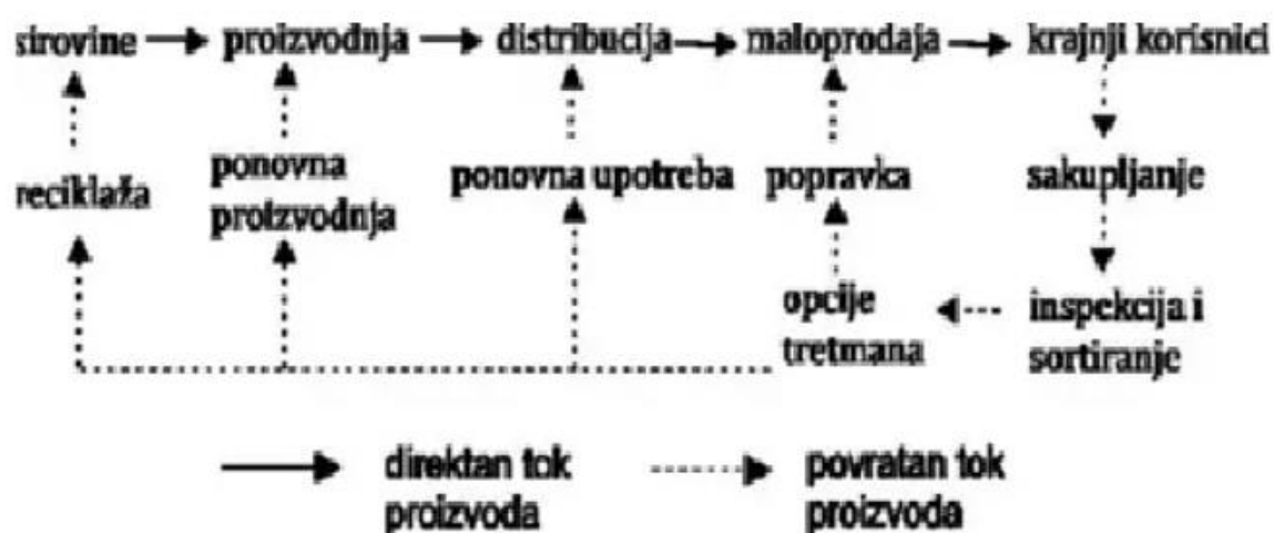
Slika 8. Pojednostavljena shema aktivnosti povratne logistike [19]
