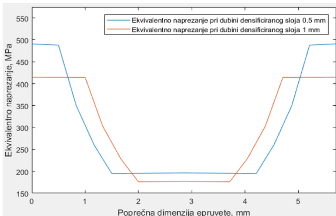
Slika 69. Usporedba ekvivalentnih napreznaja po poprečnom presjeku kod elastoplastičnog ponašanja materijala epruvete za različite dubine densifikacije
