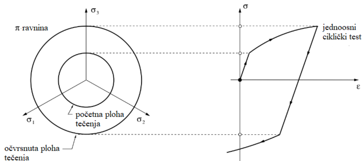
Slika 23. Izotropno očvršćenje [11]
