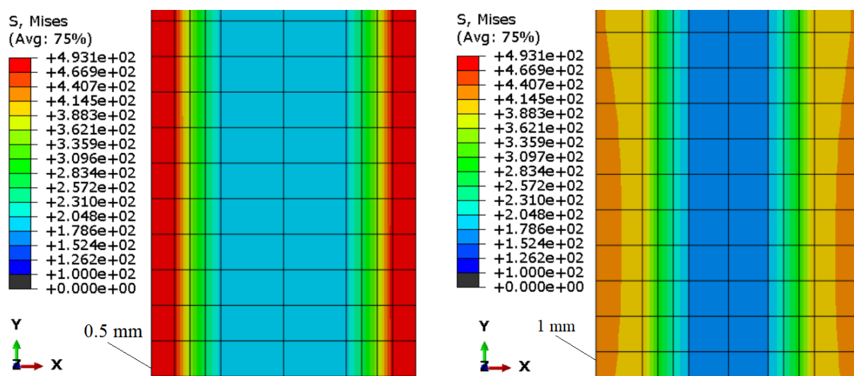
Slika 68. Usporedba ekvivalentnih napreznaja na sredini ispitnog dijela epruvete
