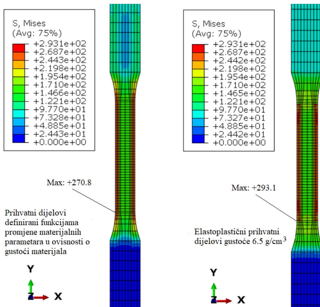
Slika 65. Usporedba ekvivalentnih napreznja ovisno o konstitutivnom ponašanju prihvatnog dijela epruvete
