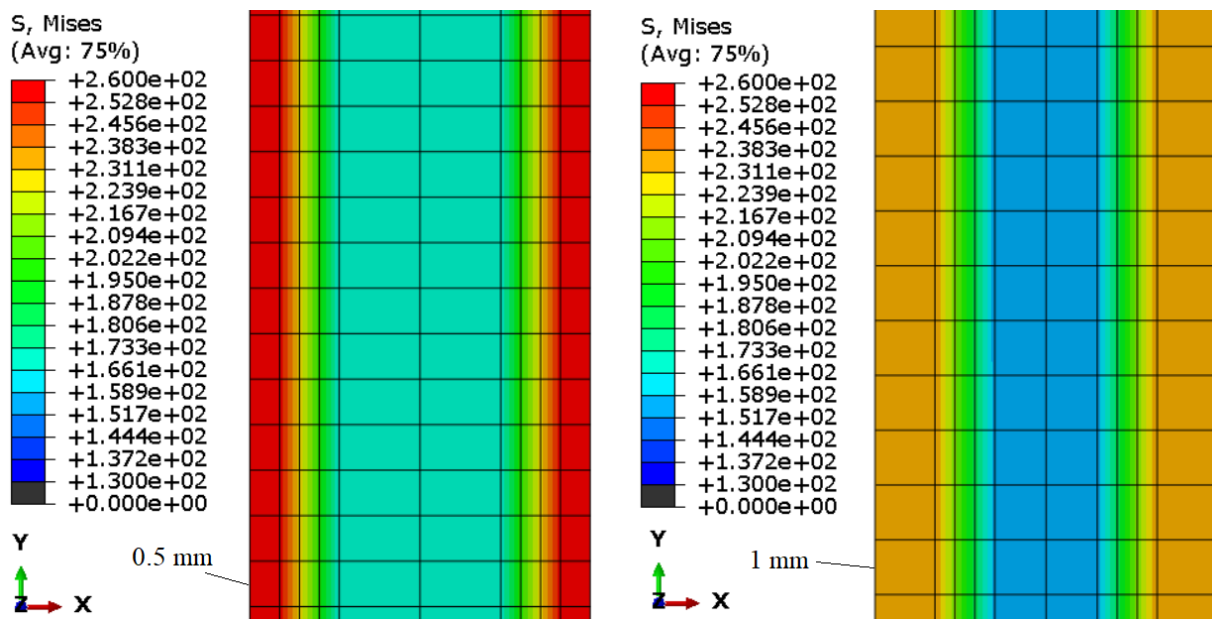
Slika 58. Usporedba ekvivalentnih napreznanja na sredini ispitnog dijela epruvete za različite dubine densifikacije
