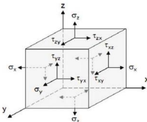
Slika 16. Tenzor naprezanja [13]
