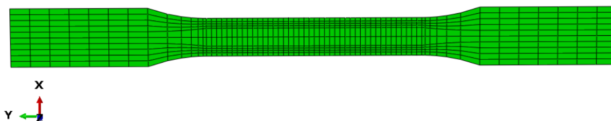
Slika 54. Optimalna mreža
