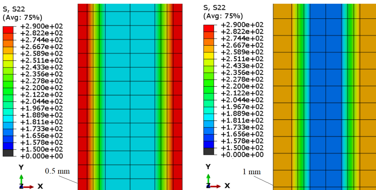
Slika 59. Usporedba napreznanja u smjeru osi y na sredini ispitnog dijela epruvete za različite dubine densifikacije
