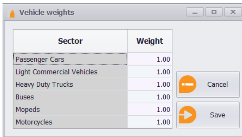
Slika 2.6. PCU weights
