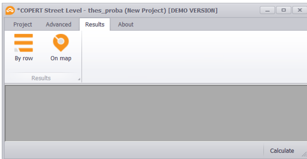
Slika 2.8. Izbornik Results
