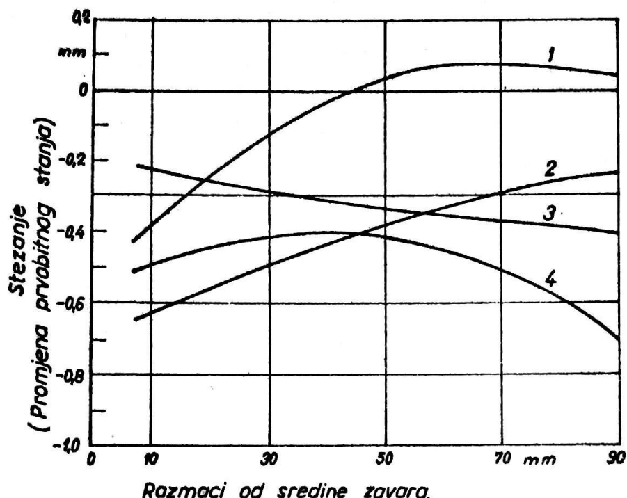
Slika 10. Utjecaj postupka zavarivanja konstrukcijskog čelika na veličinu uzdužne deformacije [6]
