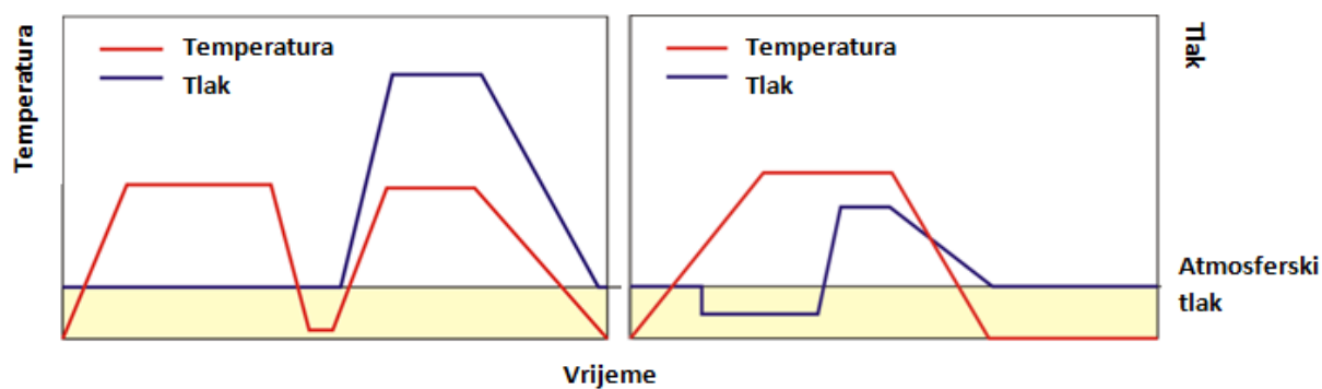
Slika 2.24 Dijagrami temperatura-tlak-vrijeme različitih sinter HIP postupaka: a) sinter+HIP; b) sinter/HIP [59]
