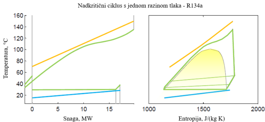
Slika 9. T-Q i T-s dijagrame za nadkritični ciklus u kojem je radni fluid R134a [2]
