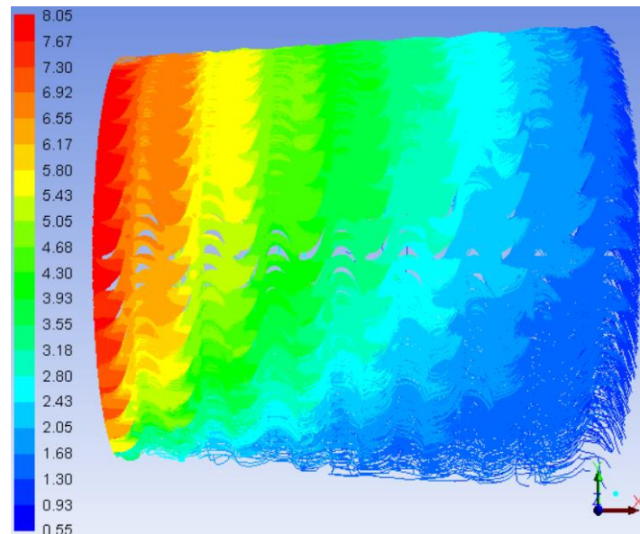
Slika 65. Rezultati numeričkih simulacija strujanja u maloj ORC turbini
