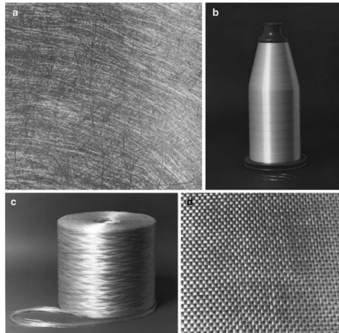
Slika 8. Mogući oblici staklenih vlakana [4]
