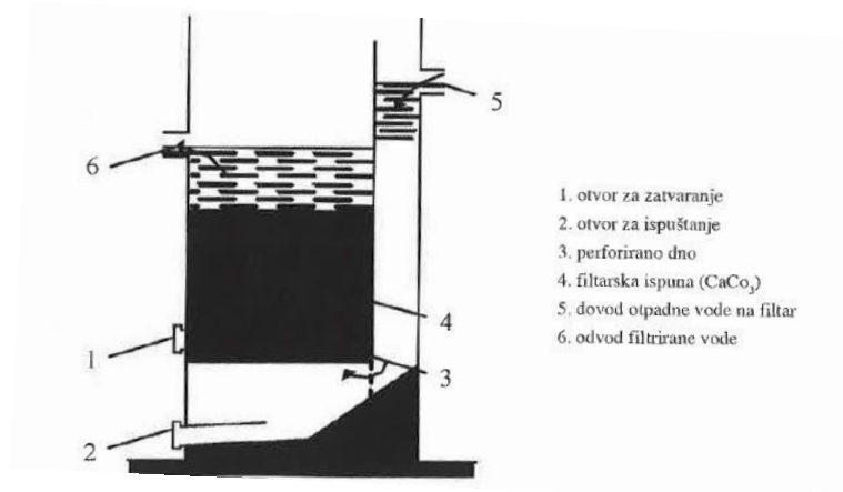
Slika 9. Neutralizacija na filtarnom sloju vapnenca [8]
