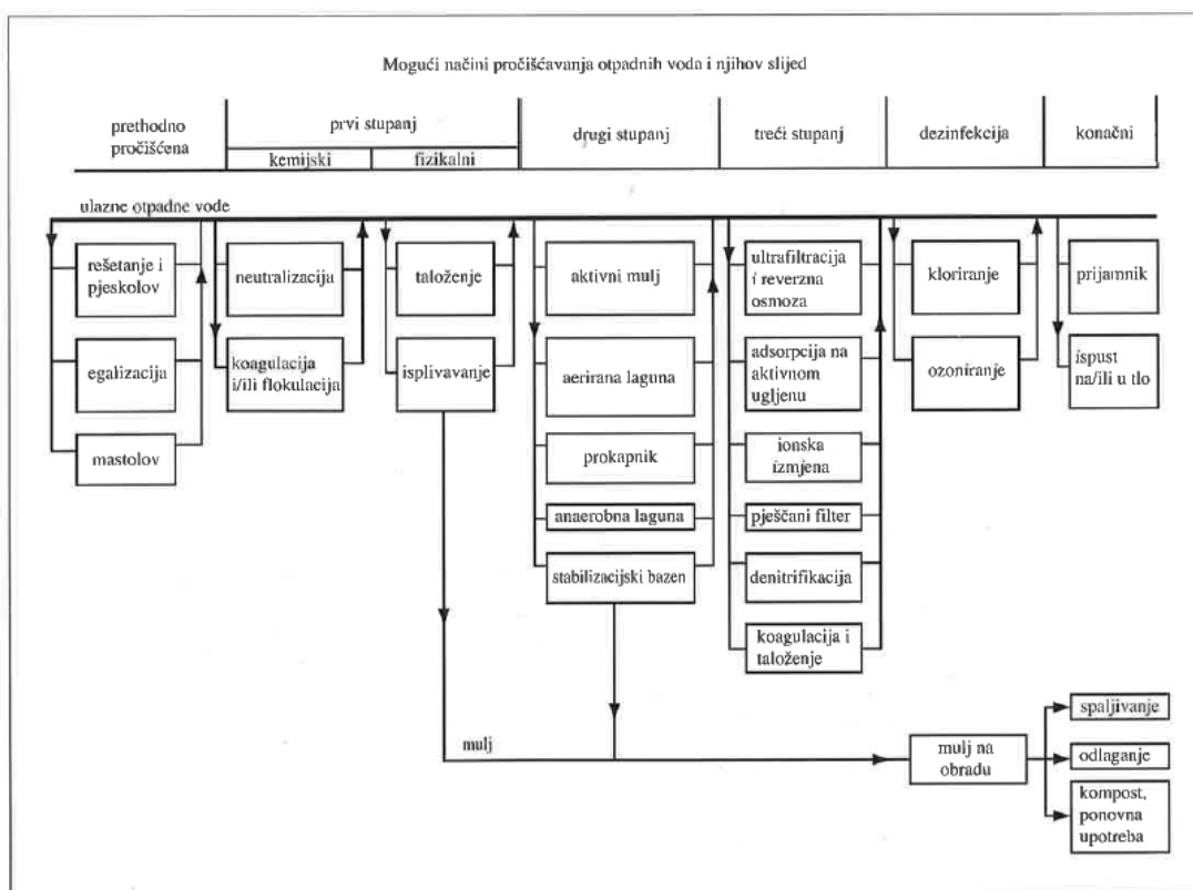
Slika 7. Dijelovi tehnološke linije pročišćavanja otpadnih voda [8]
