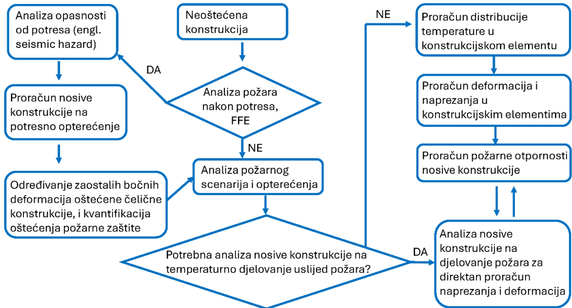
Slika 6 Koraci u FFE analizi ponašanja okvirnih konstrukcija [25]
