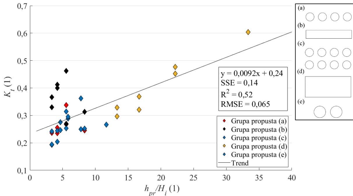
Slika 73 Odnos dubine unutar propust ( h_{pr} ) i valne visine incidentnog vala ( H_i ) naspram srednjeg koeficijentu tranmisije unutar mjernog područja ( K_t ) (Slika 63) za pojedine testove provedene u okviru numeričkog modeliranja djelomično uronjene grupe propusta (W2) (Tablica 10); u prirodnom mjerilu
