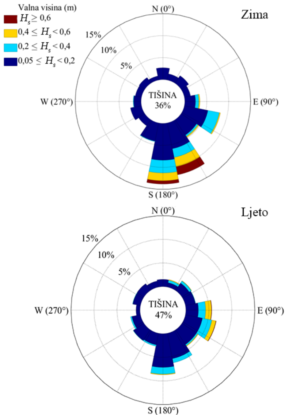
Slika 52 Ruže valova temeljene na mjerenjima provedenim pomoću ADCP 1 koji se nalazi ispred propusta tijekom zimskog (15. 2. 2017. - 31. 3. 2017.) i ljetnog razdoblja (4. 7. 2017. - 31. 8. 2017.); izvedene ruže odnose se na satno osrednjene vrijednosti valnih visina
