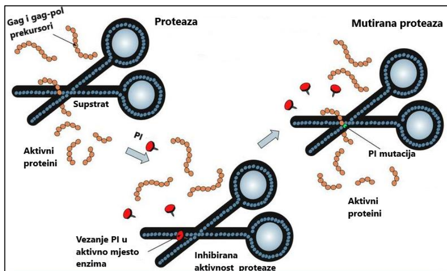
Slika 11. Mehanizam razvoja rezistencije na PI promjenom ključnih aminokiselina u aktivnom mjestu PR. Preuzeto i prilagođeno: https://www.immunopaedia.org.za/treatment-diagnostics/hiv-infection-treatment/arv-mode-of-action/ .
