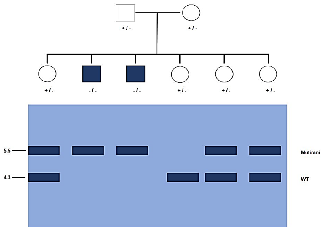
Slika 27. Na gornjem dijelu je shematski prikazan rodovnik križanja dva heterozigota za disruptirani Ftz-F1 alel. Na donjem sliku je prikazan rezultat hibridizacije po Southernu. Alel divljeg tipa (WT) daje band od 4.3 kb, a mutirani od 5.5 kb.
