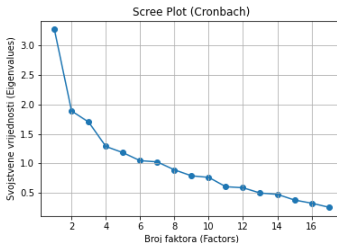
Slika 3. Odnos faktora i pripadajućih svojstvenih vrijednosti za Cronbach podskup podataka
