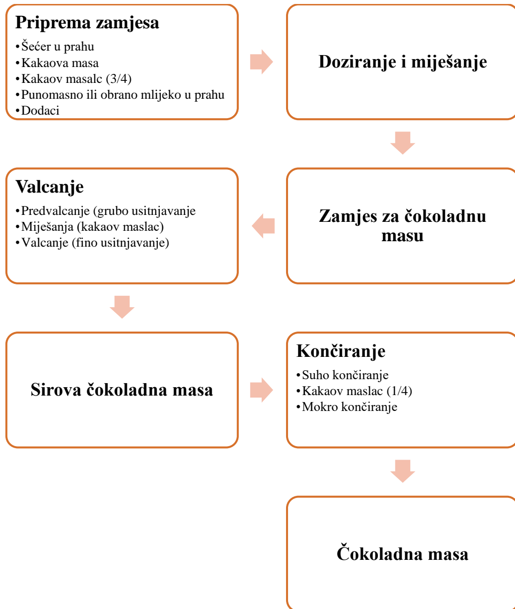
Slika 4. Shema tehnoloških operacija u izradi čokoladne mase konvencionalnim postupkom (Goldoni, 2004)
