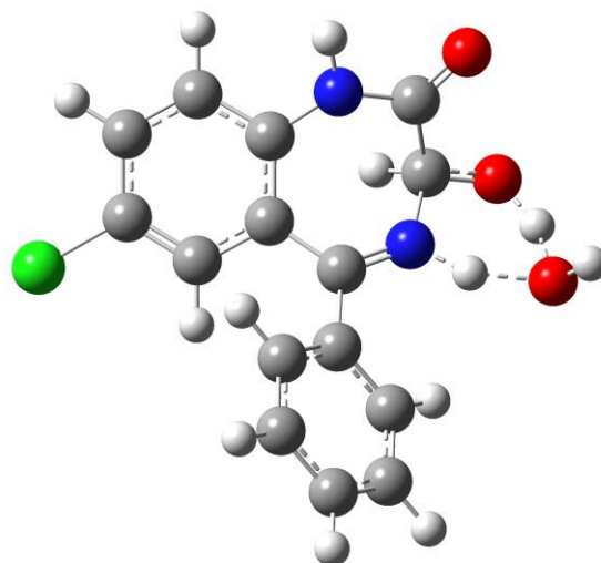
Slika 14. Struktura prijelaznog stanja adicije imina N4 na karbonilnu skupinu C3=O u aldehidu i formiranje (3R)-oksazepama ( TS_{ald} ). Struktura je optimizirana na B3LYP/6-31+G(d) razini s jednom eksplicitnom molekulom vode [ NImag/(cm^{-1}) = 1 (1159.48i)].
