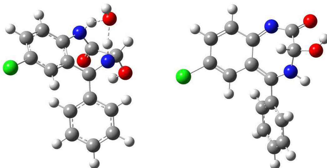
Slika 15. Struktura prijelaznog stanja proton transfera s N1-H na N4 s jednom eksplicitnom vodom [ NImag/(cm^{-1}) = 1 (319.44i)] (lijevo) i produkt prethodno opisanog proton transfera (desno), pri čemu je vidljivo da ne dolazi do kidanja N4-C3 veze. Strukture su optimizirane na B3LYP/6-31+G(d) razini.
