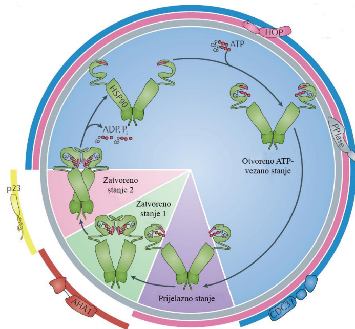
Slika 4. Shematski prikaz Hsp90 konformacijskog ciklusa i vezanja košaperona. Nakon vezanja ATP-a, Hsp90 prelazi iz otvorenog ATP-vezanog stanja u prijelazno stanje kada dolazi do zatvaranja „poklopca“. Zatim N-terminalni krajevi monomera stupaju u interakciju (zatvoreno stanje 1), te dolazi do uvijanja monomera (zatvoreno stanje 2). Različiti košaperoni se vežu na određene konformacije Hsp90: HOP stabilizira otvorenu konformaciju i tako inhibira ATP-aznu aktivnost, PPIase se vežu na sva konformacijska stanja Hsp90, CDC37 se veže rano u ciklusu i važan je za vezanje klijenata kinaza, AHA1 posreduje formaciju zatvorenog stanja 1, a p23 stabilizira zatvoreno stanje 2 (preuzeto i prilagođeno iz Schopf i sur., 2017).
