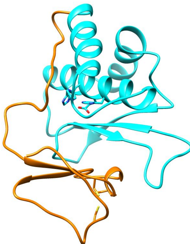
Slika 19. Prikaz predikcije trodimenzijske strukture domene SprT humanog proteina ACRC dobivenog programom Modeller . 36
