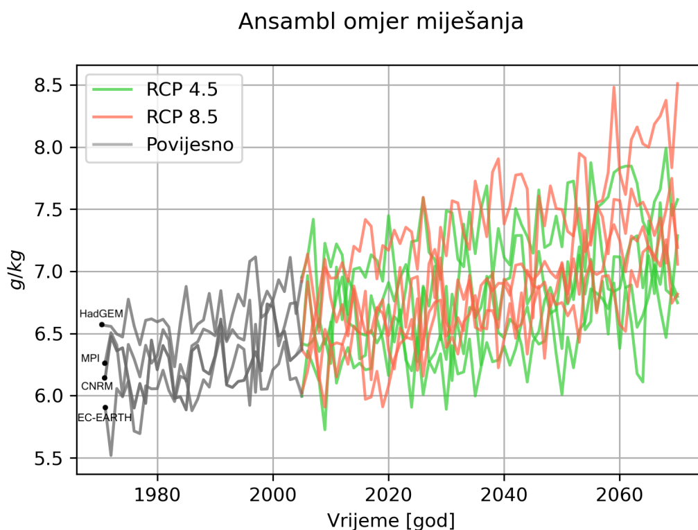
Slika 3.1.1: Ansambl omjer miješanja. Prikazan je vremenski niz godišnjih prostornih srednjaka svih vrijednosti prizemnog omjera miješanja. Svaki globalni model je za svaki scenarij prikazan zasebno i označen je na grafu. Sivo obojene krivulje prikazuju povijesne klime, dok zelene i crvene krivulje scenarije RCP 4.5 i RCP 8.5.
