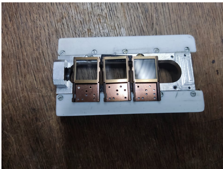
Slika 3.6: Držač u staroj mikroprobi. Prikazano je postavljanje dozimetara i prazno mjesto pored njih koje je služilo mjerenju toka snopa.
