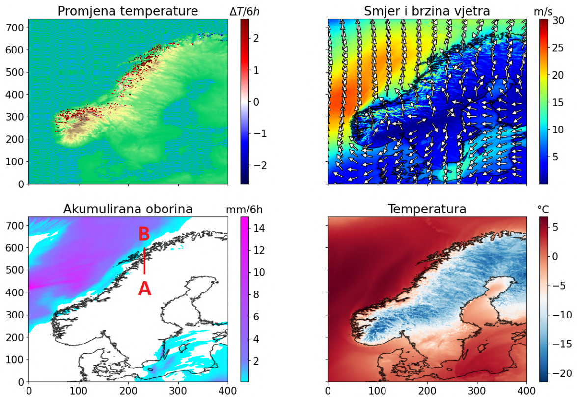
Slika 3.7. Termin s najvećim brojem ZO-a u C poddomeni za CT 5 (20. 1. 1998., 12 UTC). Prikazani su orografija i lokacije i iznosi promjene temperature (gore lijevo), smjer (vektori) i brzina (boja) vjetra (gore desno), akumulirana 6-satna oborina (dolje lijevo) i temperatura na 2 m (dolje desno). Crvena linija na slici oborine pokazuje položaj vertikalnog presjeka prikazanog na slici 3.8
