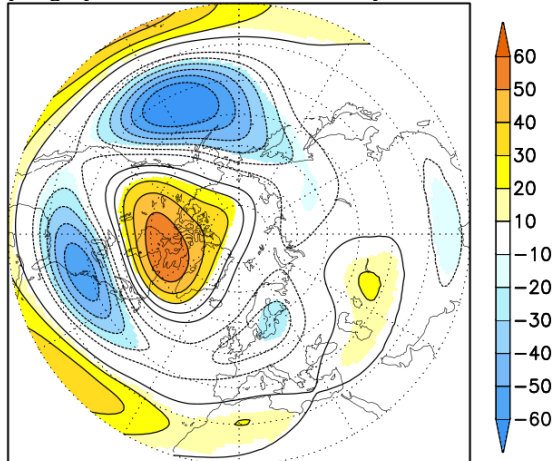
(e) regr (Niño 3.4, 20CRV3 GH200) 1930-1959
