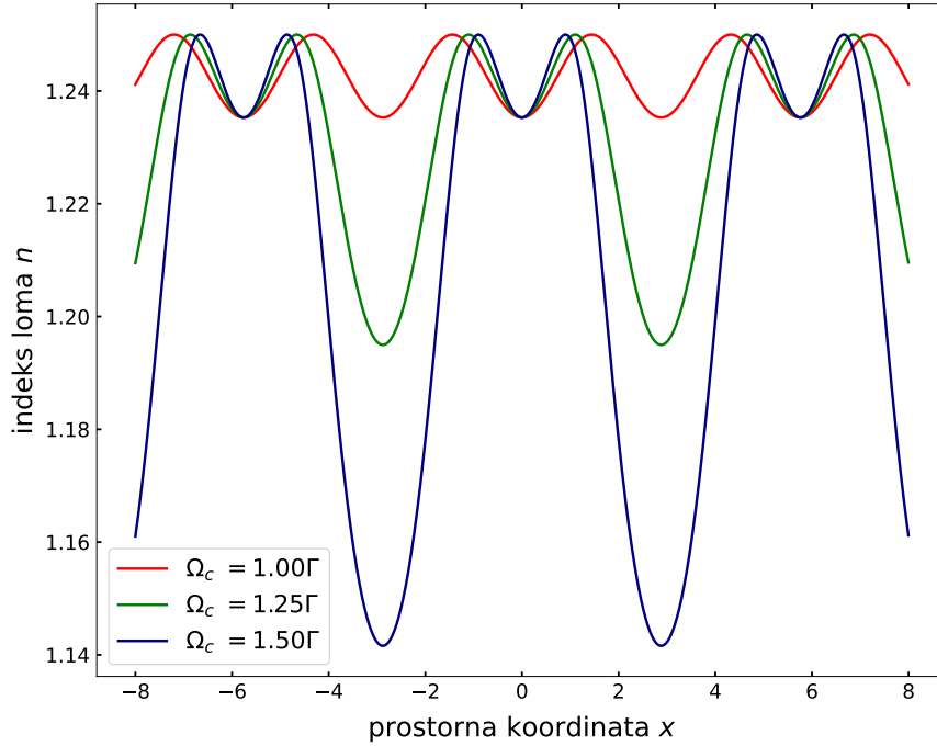
Slika 2.10: Prostorna promjena indeksa loma n za tri različite vrijednosti parametra Rabijeve frekvencije \Omega_c uz ostale parametre \Gamma = 0,5 , \gamma = 0,5\Gamma , \Omega_p = 0,001\Gamma , \Delta_c = -1 i \Delta_p = -1 . Grafički prikaz izrađen je korištenjem izraza 2.56.
