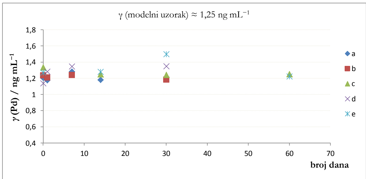
Slika 19. Stabilnost modelnih uzoraka paladija na kvarecnim filtrima, a) 5 % \text{HNO}_3 (v/v), b) 5 % \text{HNO}_3 / 1 % \text{HCl} (v/v), c) 5 % \text{HNO}_3 / 2 % \text{HCl} (v/v), d) 5 % \text{HNO}_3 / 5 % \text{HCl} (v/v) i e) 1 % \text{HCl} (v/v)
