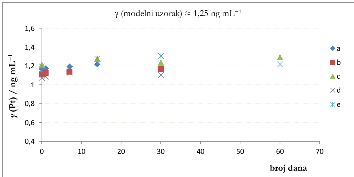
Slika 18. Stabilnost modelnih uzoraka platine na kvarecnim filtrima, a) 5 % \text{HNO}_3 (v/v), b) 5 % \text{HNO}_3 / 1 % \text{HCl} (v/v), c) 5 % \text{HNO}_3 / 2 % \text{HCl} (v/v), d) 5 % \text{HNO}_3 / 5 % \text{HCl} (v/v) i e) 1 % \text{HCl} (v/v)
