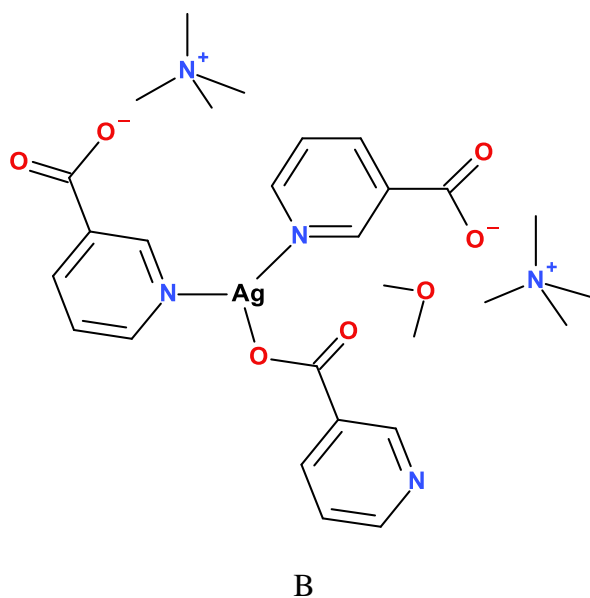
Slika 18. Koordinacijsko okruženje oko iona srebra(I) kod spojeva A) catena- \{[piridin-3\text{-karboksilato-(O,O')}]srebra(I)\} i B) amonijeva bis[piridin-3-karboksilato-(O,N,N')] argentata(I) monohidrata.
