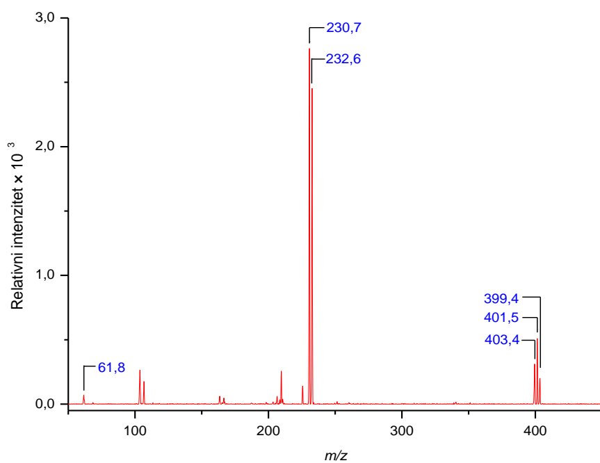
Slika D6. A) ESI + -MS i B) ESI - -MS spektri kompleksa [Ag(NO_3)(3-Ipy)_2]^+ , K6 .
