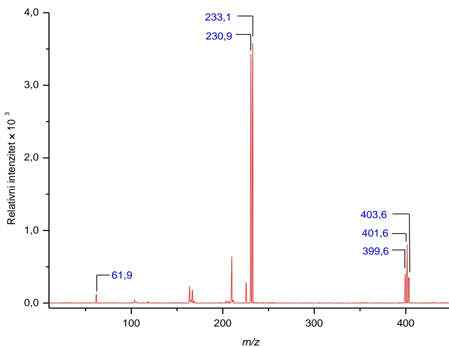
Slika D7. A) ESI + -MS i B) ESI - -MS spektri kompleksa [Ag(NO_3)(2,5-Cl_2py)_2] , K7 .
