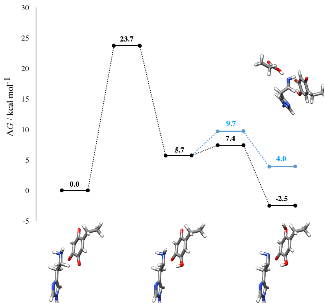
Slika 41. Profil za reakciju oksidativne deaminacije histamina koja je katalizirana enzimom DAO u okviru QM-klastera pristupa s ispitanim alternativnim prijenosom protona iz amino skupine histamina na kisik karboksilne skupine iz bočnog ogranka Asp373 u drugom koraku reakcije. Zbog preglednosti slike prikazane su samo one vrste koje direktno sudjeluju u reakciji.
