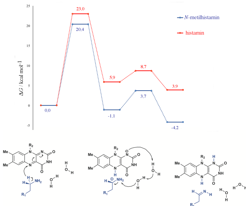
Slika 27. Profili za reakciju oksidativne deaminacije histamina (crveno) i N -metilhistamina (plavo) kataliziranu enzimom MAO B u okviru pristupa QM-klastera.
