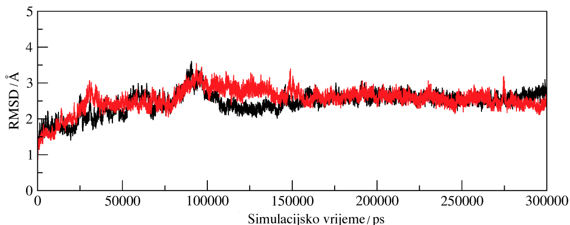
Slika 22. Vrijednosti RMSD za enzim MAO B u kompleksu s monokationima HIS (crveno) i NMH (crno) tijekom 300 ns molekulsko-dinamičkih simulacija.
