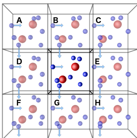
Slika 15. Shematski prikaz periodičnih rubnih uvjeta koji se koriste u molekulsko-dinamičkim simulacijama.
