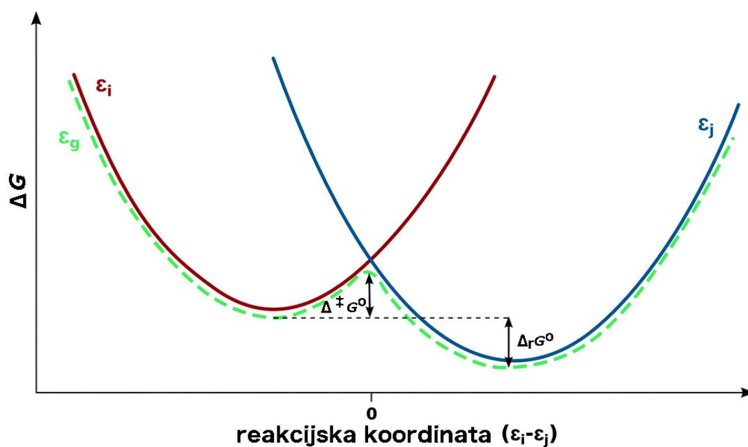
Slika 17. Shematski prikaz metode EVB, gdje su \varepsilon_i i \varepsilon_j energije dva dijabatska stanja, \Delta^\ddagger G^0 je standardna Gibbsova energija aktivacije za danu reakciju, \Delta_r G^0 je standardna Gibbsova energija reakcije. Reakcijska koordinata je predstavljena razlikom energije dva dijabatska stanja ( \varepsilon_i - \varepsilon_j ). Preuzeto i prerađeno iz 120 .
