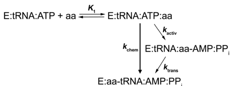
Slika 4.10 Mehanizam aminoaciliranja. Minimalna shema reakcije aminoaciliranja u kojoj je vezanje aminokiseline u brzoj ravnoteži. Maksimalni koeficijent brzine aminoaciliranja u uvjetima jednog obrtaja enzima sastavljen je od pojedinačnih koeficijenata aktivacije ( k_{activ} ) i prijenosa ( k_{trans} ). Preuzeto i prilagođeno iz Cvetesic i sur. 2014 134 .
