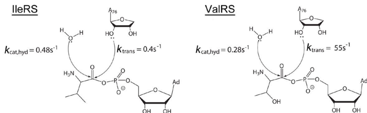
Slika 2.10 Kinetička razdioba Val-AMP i Thr-AMP u sintetskom mjestu IleRS odnosno ValRS. k_{trans} -koeficijent brzine prijenosa aminokiseline, k_{cat, hyd} – koeficijent brzine hidrolize aminoacil-adenilata u ustaljenom stanju. Preuzeto i prilagođeno iz Dulic i sur. 2010 11 .
