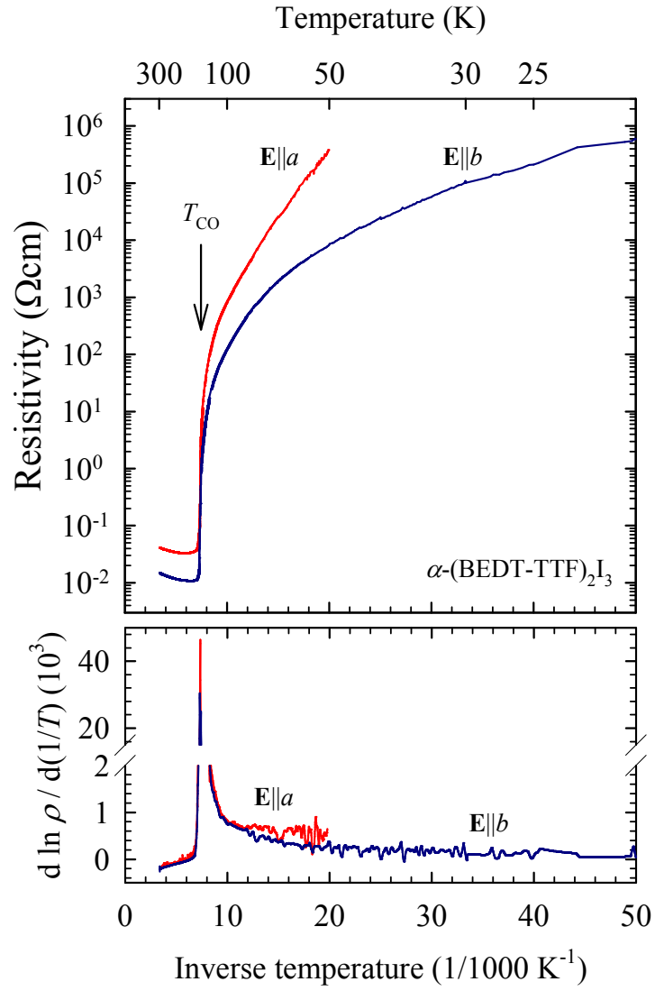
Slika 8.21 – Otpornost (gornji panel) i logaritamska derivacija otpora (donji panel) \alpha -(BEDT-TTF) _2 I _3 u ovisnosti o inverznoj temperaturi za \mathbf{E} \parallel a (crvena linija) i \mathbf{E} \parallel b (plava linija).
