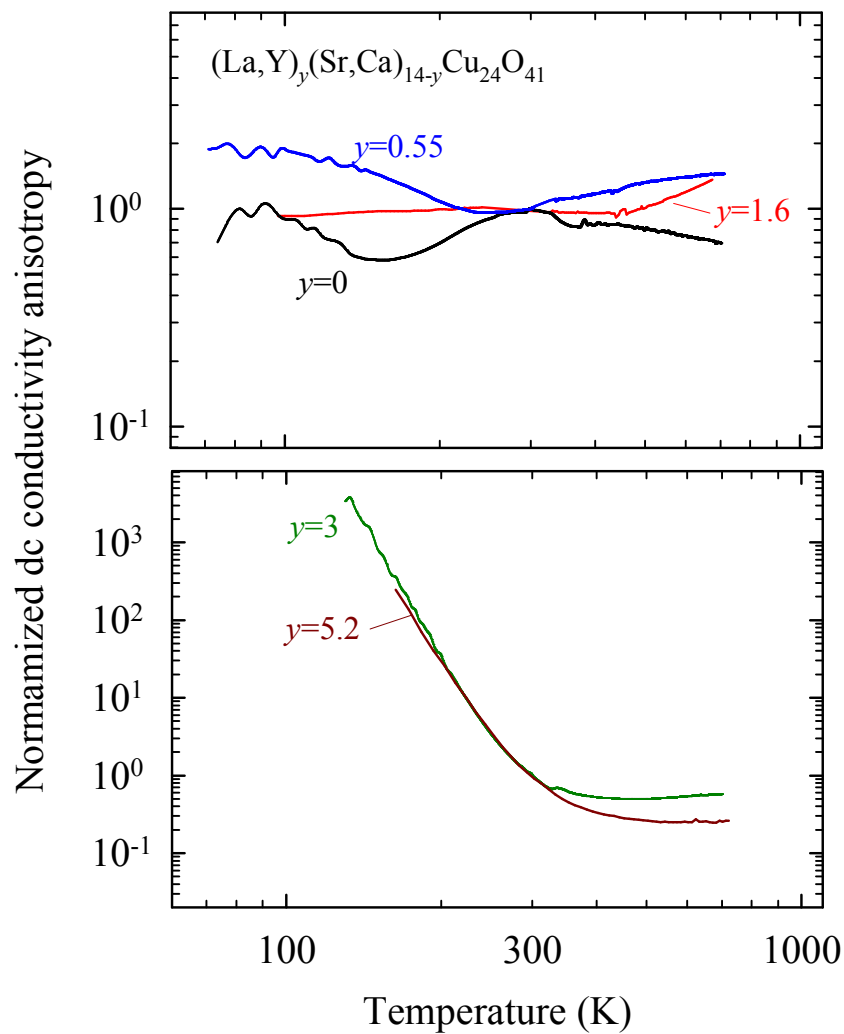
Slika 8.7 – Temperaturna ovisnost anizotropije vodljivosti (\text{La}, \text{Y}, \text{Sr}, \text{Ca})_{14}\text{Cu}_{24}\text{O}_{41} za razne sadržaje La/Y y normalizirane na vrijednost na sobnoj temperaturi.
