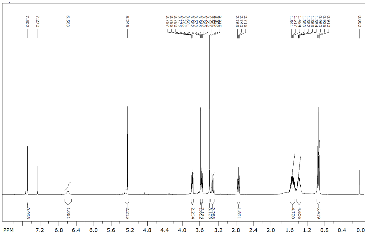
Slika D2.6. 1H NMR spektar produkta amida N -butil-2,5,7-trioksa-8-azadec-8-en-10-amida 5
