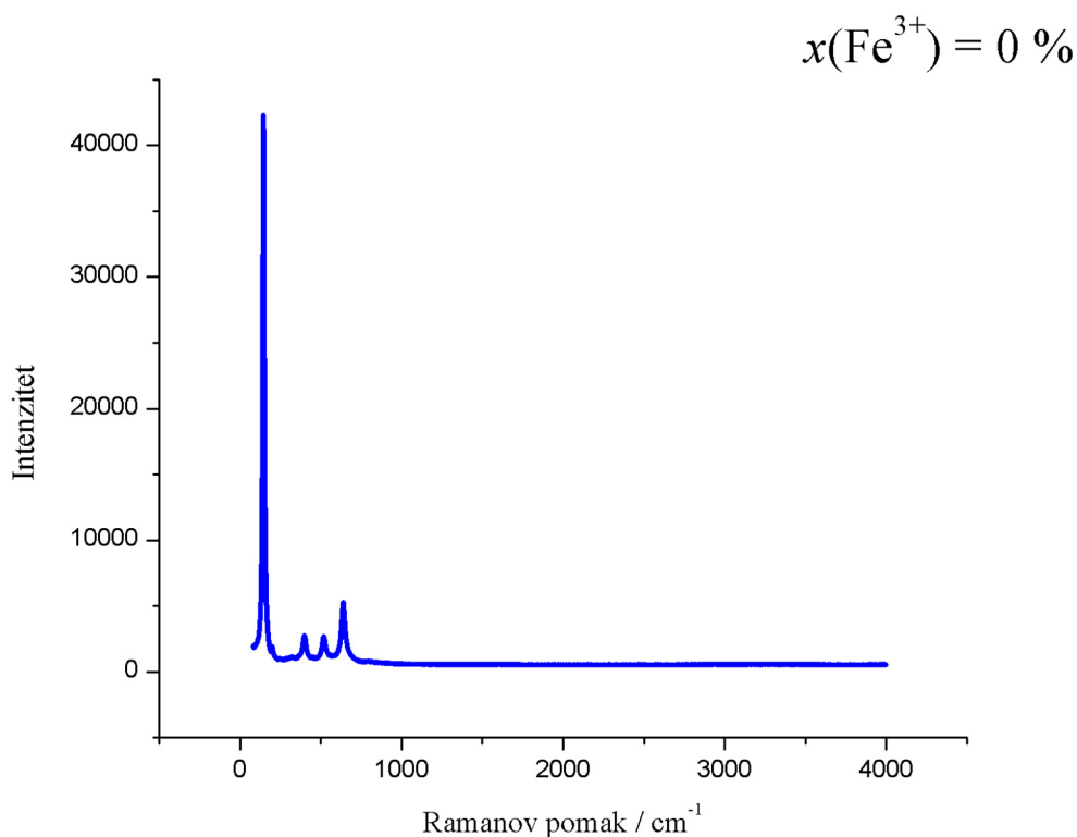
Slika 18. Ramanov spektar uzorka \text{TiFe}_0 u području do 4000 \text{ cm}^{-1}
