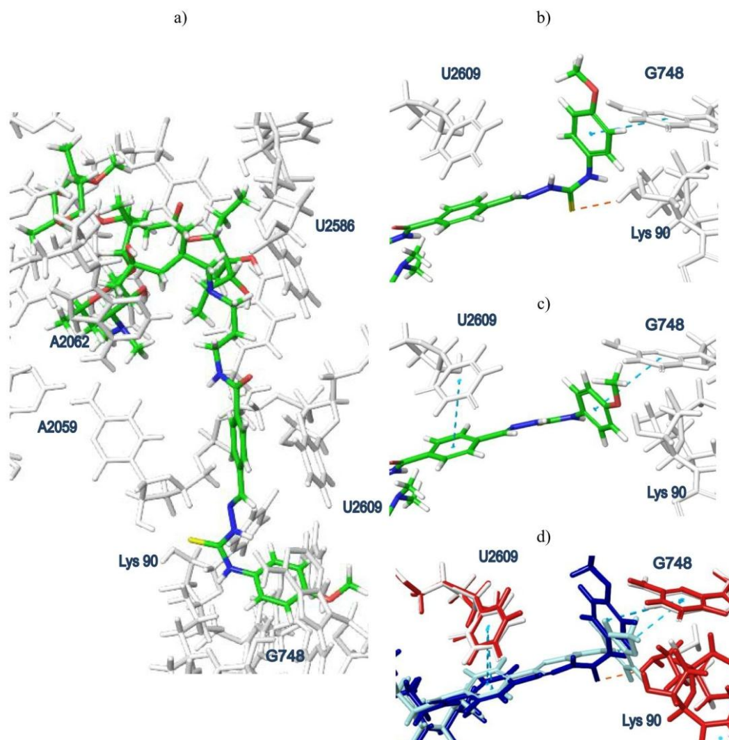
Slika 15. Rezultati Monte Carlo konformacijske pretrage liganda E u PTAR-u ribosoma bakterije Escherichia coli : a) geometrija energetski najpovoljnijeg konformera, b) nekovalentne interakcije energetski najpovoljnijeg konformera s nukleotidom G748 i aminokiselinom Lys 90, c) nekovalentne interakcije između konformera koji ima 4,30 kJ mol -1 nepovoljniju energiju od najpovoljnijeg konformera i nukleotida G748 i U2609, d) usporedba nekovalentnih veza koje ligand tvori s nukleotidima G748 i U2609 te aminokiselinom Lys 90. Tamno plava i crvena boja označava konformaciju prikazanu na slici 15b, a svjetlo plava i bijela onu prikazanu na slici 15c.
