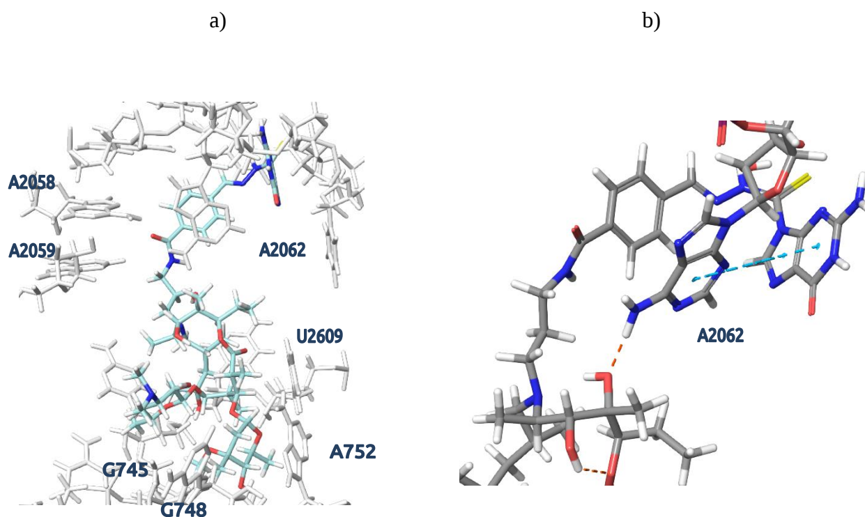
Slika 20. Najpovoljniji oblik vezanja izračunat Monte Carlo simulacijom konformera liganda M kojem je energija 4,3 \text{ kJ mol}^{-1} veća od najpovoljnijeg konformera izračunatog metodom molekulskog uklapanja a) vezanje u PTAR ribosoma bakterije Escherichia coli b) nekovalentne veze s nukleotidom A2062. Na slici a nukleotidi i aminokiseline ribosoma bakterije Escherichia coli su prikazani bijelom bojom.
