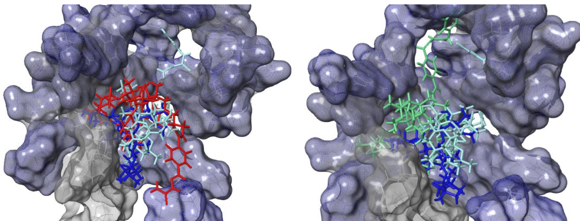
Slika 11. Usporedba vezanja liganada B, C, D i azitromicina u vezno mjesto PTAR-a bakterije Escherichia coli izračunata metodom Monte Carlo (ligand B, azitromicin) i molekulskog uklapanja (ligand C i ligand D). Azitromicin je prikazan tamnoplavom, ligand B crvenom, ligand C zelenom i ligand D svijetloplavom bojom. Orijentacija veznog mjesta ista je na lijevoj i desnoj slici.
