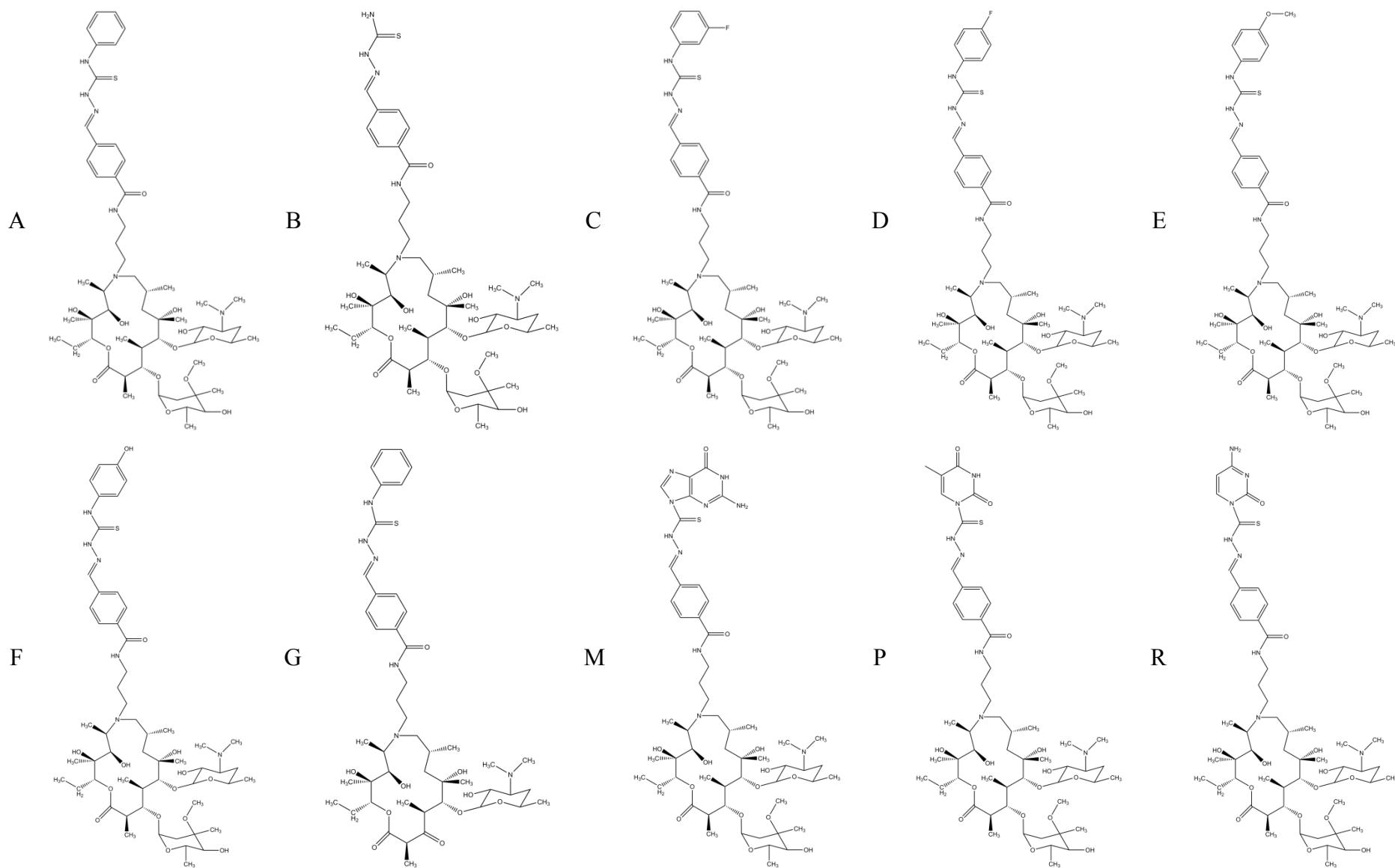
Slika 3. Dvodimenzionalni prikaz struktura liganada koji su korišteni tijekom računalnog istraživanja.
