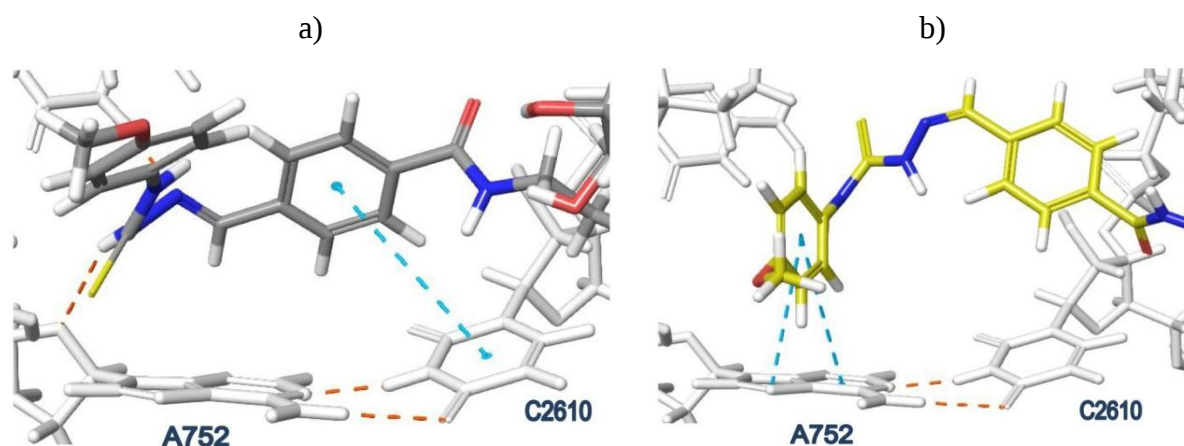
Slika 14. Rezultati molekuskog uklapanja liganda E u PTAR ribosoma bakterije Escherichia coli a) nekovalentne interakcije između konformera najmanje energije te nukleotida C2610 i A752 23S rRNA, b) nekovalentne interakcije između konformera koji ima 1,80 kJ mol -1 nepovoljniju energiju od najpovoljnijeg konformera i nukleotida A752. Nukleotidi i aminokiseline ribosoma bakterije Escherichia coli su prikazani bijelom bojom.
