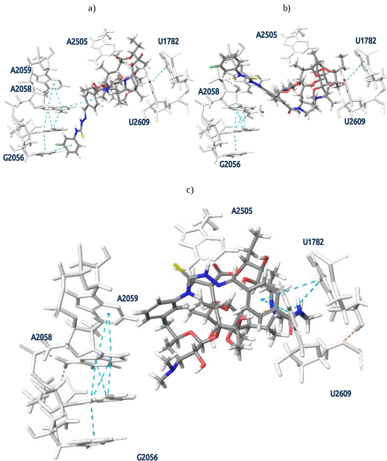
Slika 22. Konformeri najmanje energije dobiveni Monte Carlo simulacijama konformera liganda C* u PTAR-u ribosoma bakterije Escherichia coli a) gdje se na poziciji 2058 23S rRNA nalazi nemetilirani adenin b) gdje se na poziciji 2058 23S rRNA nalazi dimetilirani adenin c) gdje se na poziciji 2058 23S rRNA nalazi gvanin. Nukleotidi i aminokiseline ribosoma bakterije Escherichia coli su prikazani bijelom bojom.
