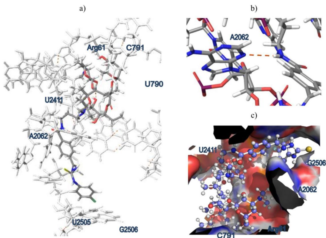
Slika 10. Vezanja liganda D u PTAR bakterije Escherichia coli : a) energetski najpovoljniji način pronađen metodom molekuskog uklapanja, b) vodikova veza koju ligand tvori s A2062 kod energetski najpovoljnijeg načina vezanja pronađenog metodom molekuskog uklapanja, c) vezanje energetski najpovoljnijeg konformera dobivenog molekulskim uklapanjem liganda u PTAR ribosoma bakterije Escherichia coli . Na slici a) nukleotidi i aminokiseline ribosoma bakterije Escherichia coli su prikazani bijelom bojom.
