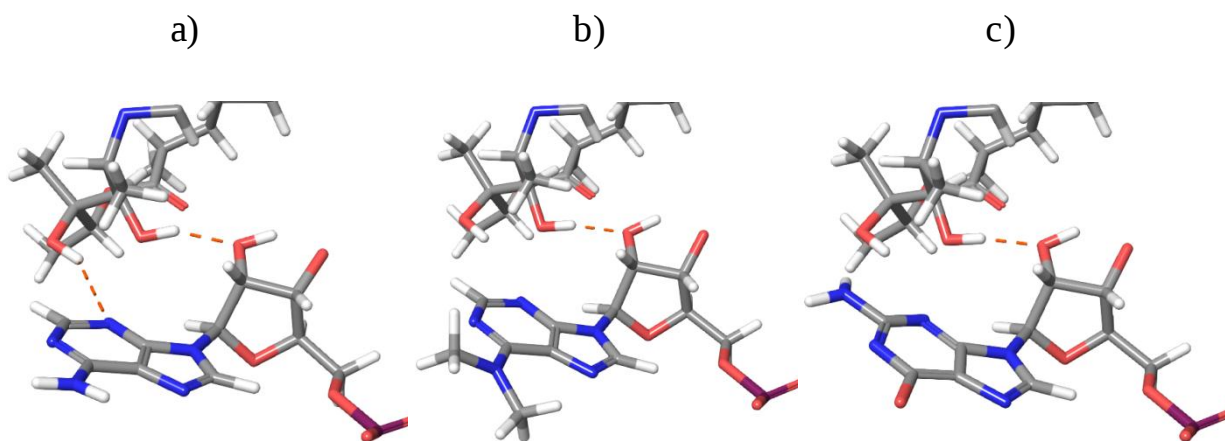
Slika 21. Monte Carlo simulacija liganda A* u PTAR-u ribosoma bakterije Escherichia coli a) gdje se na poziciji 2058 23S rRNA nalazi adenin a kao početna struktura je korišten konformer najniže energije dobiven metodom molekuskog uklapanja b) gdje se na poziciji 2058 23S rRNA nalazi dimetilirani adenin, a kao početna struktura je korišten konformer najniže energije dobiven Monte Carlo pretragom liganda A* u PTAR-u c) gdje se na poziciji 2058 23S rRNA nalazi gvanin a kao početna struktura je korišten konformer najniže energije dobiven Monte Carlo pretragom liganda A* u PTAR-u.
