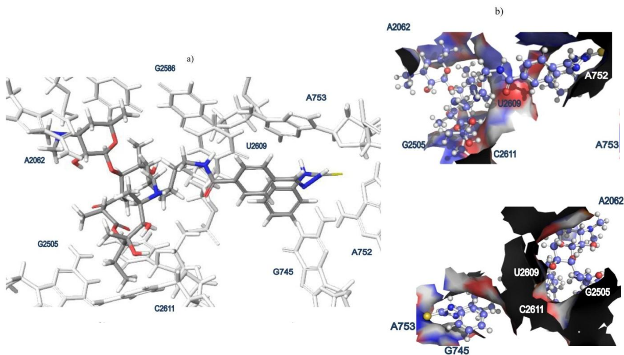
Slika 17. Rezultati molekuskog uklapanja liganda G u PTAR ribosoma bakterije Escherichia coli a) geometrija vezanja liganda G u PTAR b) položaj energetske najpovoljnijeg konformera na veznoj površini PTAR-a c) položaj energetske najpovoljnijeg konformera na veznoj površini PTAR-a i vezanje u kanal koji tvore nukleotidi A752, A753, G745 i U2609. Na slici a) nukleotidi i aminokiseline ribosoma bakterije Escherichia coli su prikazani bijelom bojom.
