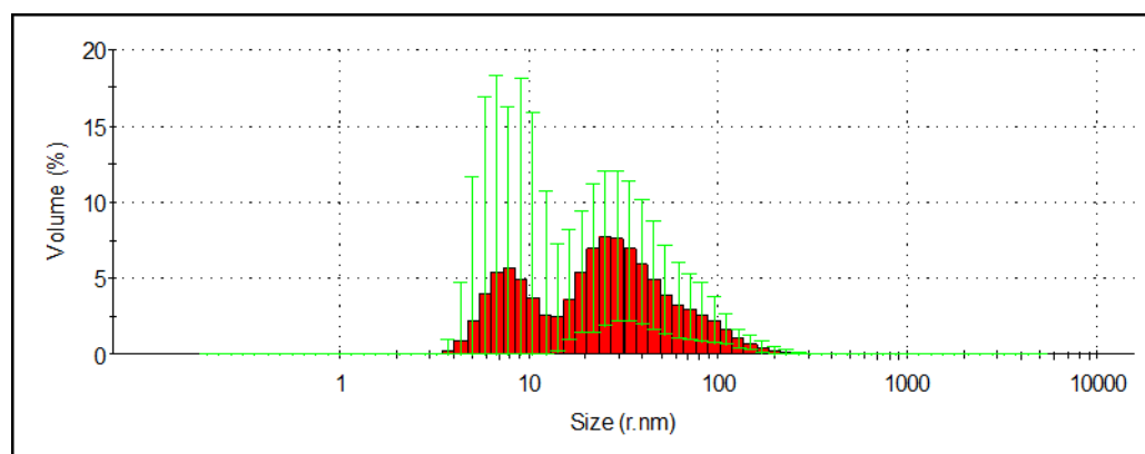
Slika 2. Prikaz distribucije veličina čestica AgNP stabiliziranih s citratnim omotačem, dobiven mjerenjem metodom dinamičkog raspršenja svjetla (DLS) (preuzeto iz Cvjetko i sur. 2018).
