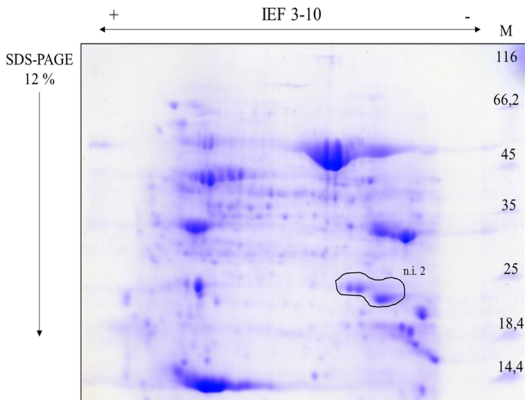
Slika 66. Ukupni toplivi proteini klijanaca duhana (kontrola) razdvojeni 2-DE. Gel je obojan bojom CBB i obrađen računalnim programom Image Master 2D Platinum . M – biljezi molekularnih masa (kDa), IEF pI 3-10 – relativan položaj proteina na gelu u odnosu na vrijednost njihove izoelektrične točke, SDS-PAGE 12% – relativan položaj proteina na gelu u odnosu na njihove mase. Kratica n.i. – nije identificiran.
