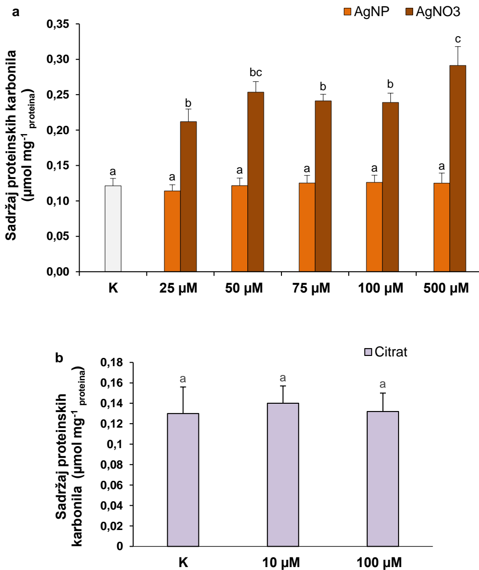
Slika 17. Sadržaj proteinskih karbonila u korijenju odraslih biljaka duhana. Biljke su tretirane sedam dana u vodenim otopinama a) AgNP i AgNO 3 , te b) citrata. Rezultati prikazani stupcima predstavljaju srednje vrijednosti od šest replika \pm standardna pogreška. Stupci označeni različitim slovima međusobno se statistički značajno razlikuju ( P \leq 0,05 ; Duncan test). K – kontrola.
