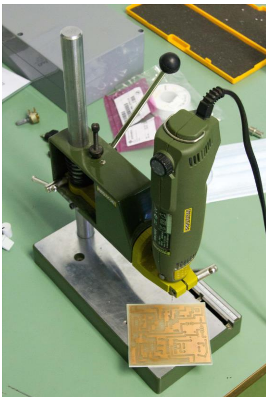
Slika 12 – Bušenje pločice
