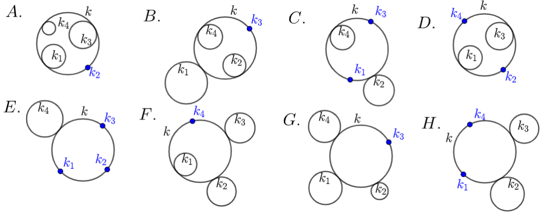
Slika 3.24.: Specijalni slučajevi Caseyevog teorema
