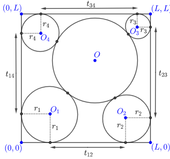
Slika 4.5.: Sangaku problem
