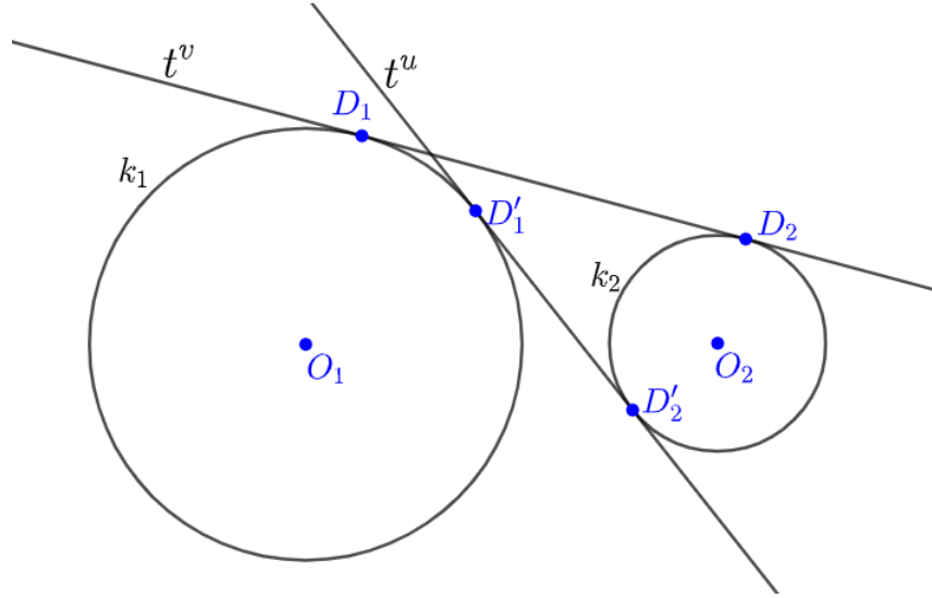
Slika 1.9.: Tangentne udaljenosti
