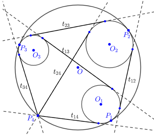
Slika 3.25.: Caseyev teorem
