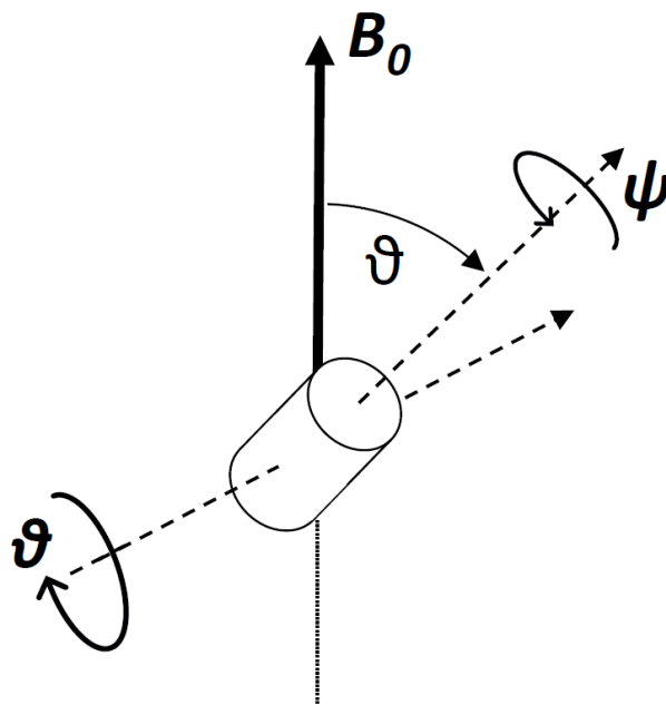
Slika 2.12: Rotacijska geometrija rotatora. Kut \vartheta je kut između osi \psi rotacije i vanjskog magnetskog polja B_0 .
