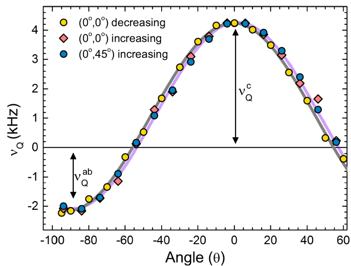
Slika 2.16: Rezultat testnog NMR mjerenja s rotatorom. Uzorak je postavljen na način da rotacija \psi ne utječe na NMR. Ponovljivost vezana uz smjer dolaska do kuta je unutar \alpha = 1^\circ .
