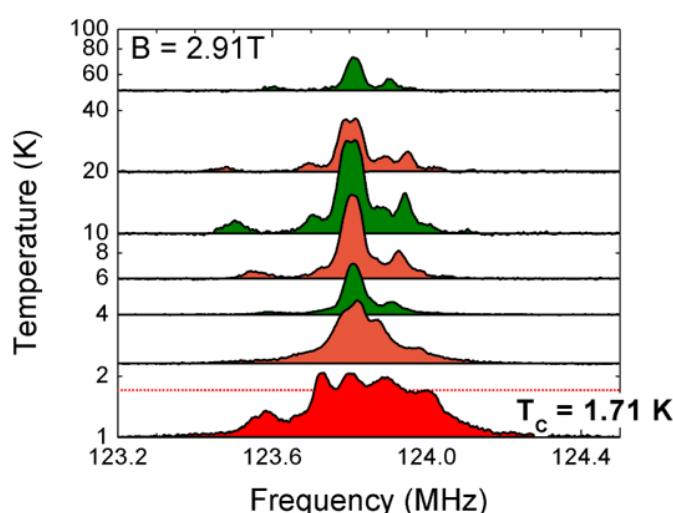
Slika 4.19: Preliminarna mjerenja NMR-a na uzorku BoNO. Širenje i pojava više linija na nižoj je temperaturi karakteristična za formiranje statičke magnetizacije u BEC fazi.
