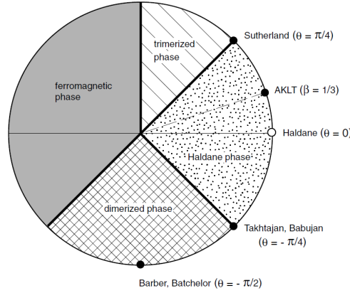
Slika 4.7: Kutna reprezentacija faznog dijagrama bilinearnog bikvadratnog hamiltonijana (jednadžba 4.6 ). Prikaz prikazuje robusnost Haldaneove faze na perturbaciju bikvadratnim članom i položaj AKLT sustava unutar Haldaneove faze. [87]
