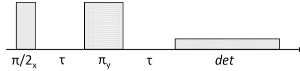
Slika 2.6: Shematski prikaz NMR sekvence Hahnove jeke. Nakon \pi/2 – pulsa slijedi vrijeme \tau nakon čega slijedi \pi puls koji rezultira rekoherencijom zbog nehomogenosti polja. Detekcija signala slijedi nakon jednako vremena \tau , kada se očekuje spinska “jeka.”
