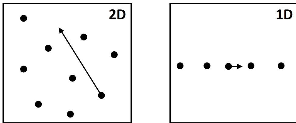
Slika 4.5: Prikaz (pojednostavljeni) problema kvazičestica u jednoj dimenziji. Dok se čestica može gotovo slobodno gibati u dvije ili više dimenzija, u jednoj dimenziji mora međudjelovati s drugim česticama.
