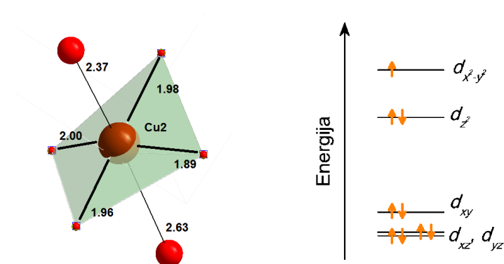
Slika 3.2: Lijevo: kisikova (crveno) okolina atoma bakra (smeđe) s pripadnim udaljenostima među atomima (izraženim u Å). Četiri su kisika bliže i tvore \text{CuO} pločicu (osjenčano). Pločica i dva vršna kisika tvore izduženi oktaedar. Desno: energije d orbitala i položaj elektrona u \text{Cu}^{2+} u okolini kisika geometrije izduženog oktaedra.
