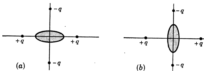
Slika 2.9: Kvadrupolni moment jezgre prikazan na klasičan način. Pozitivno nabijena jezgra orijentira se s obzirom na okolno električno polje kako bi smanjila elektrostatsku energiju. Orijentacija na (a) ima veću energiju od orijentacije na (b). Preuzeto iz [41] .
