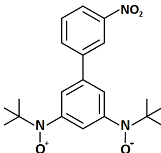
Slika 4.1: Molekula BoNO spoja. Dva slobodna elektrona koji se u molekulskoj orbitali vežu feromagnetski dolaze od dva kisika na NO granama.
