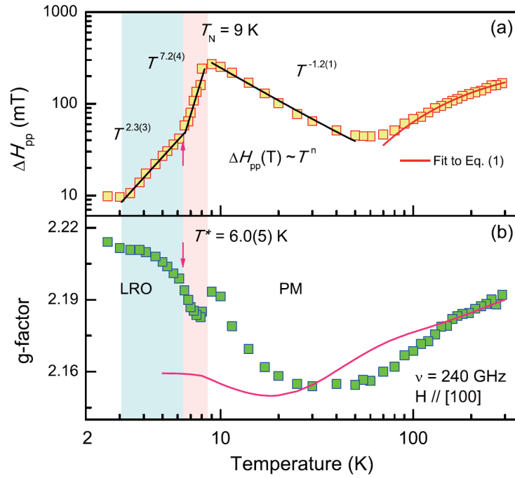
Slika 3.10: Gore: Širina EPR linije Dolje: Položaj EPR linije. Preuzeto iz [31]
