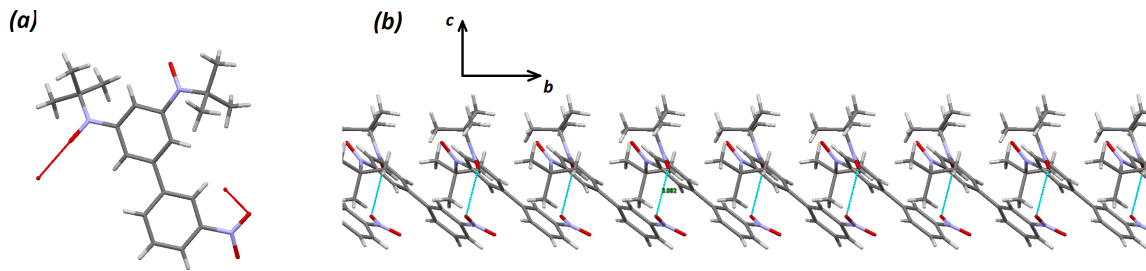
Slika 4.3: Vezanje molekula u lance. Lanac se prostire duž b kristalografske osi.
