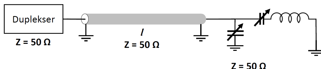
Slika 2.11: Top i bottom – tuning metode. Top tuning koristi transmisijsku liniju točno određene duljine ( \lambda/4 ) i kondenzator blizu dupleksera (“top”) kako bi postigao rezonanciju. Bottom-tuning koristi LC krug ugođene impedancije direktno kod zavojnice (“bottom”) i cijela je linija dobro ugođena.
