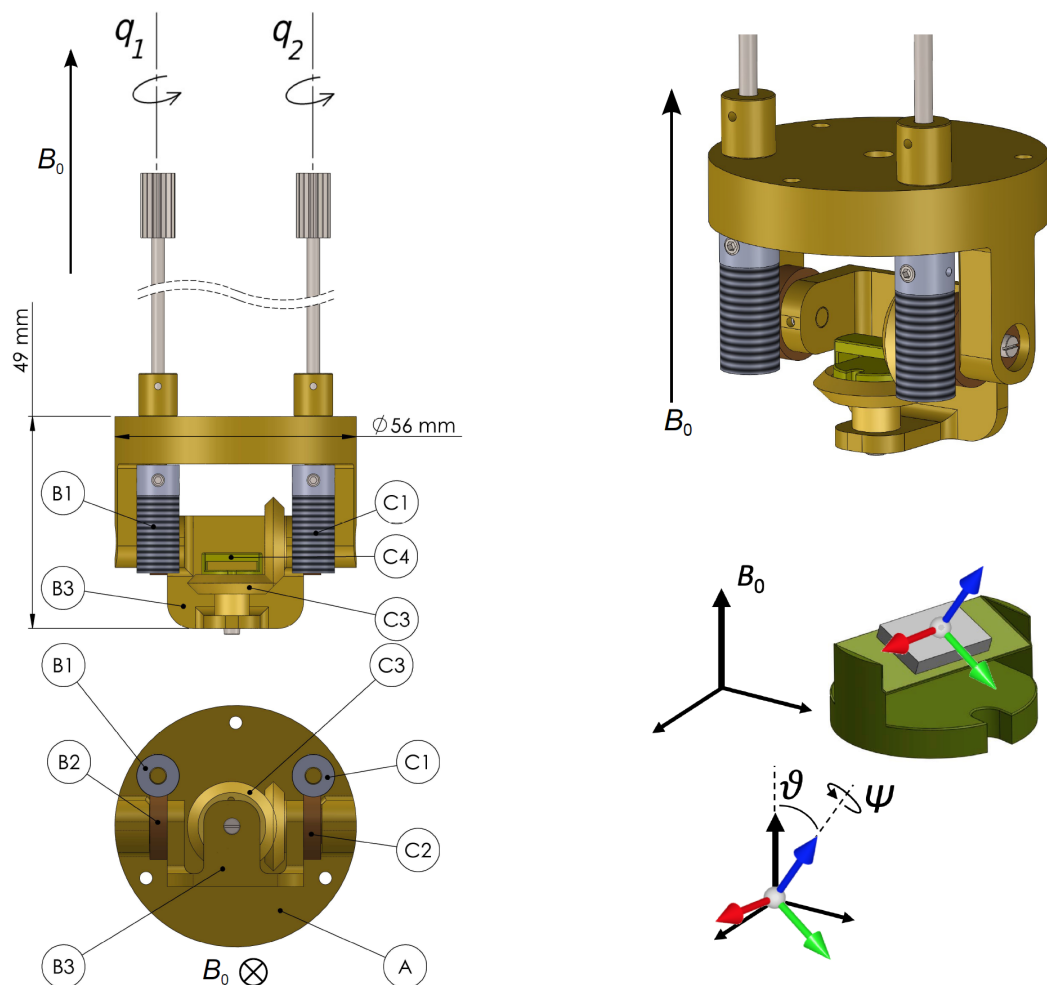
Slika 2.13: Lijevo : Nacrt dvoosnog rotatora. Naznačeni su glavni dijelovi i glavne dimenzije rotatora: A – tijelo rotatora; B1,2 – pužni vijak i kolo za u rotaciju; B3 – kolijevka čija orijentacija određuje \vartheta položaj. Služi kao nosač stožnika \psi rotacije; C1,2 – pužni vijak i kolo za v rotaciju; C3 – stožnik čija orijentacija određuje \psi rotaciju; C4 – nosač uzorka i uzorak sa zavojnicom. Naznačen je smjer vanjskog magnetskog polja B_0 na oba prikaza. Desno gore : Izometrijski prikaz rotatora. Desno dolje : Izometrijski prikaz nosača uzorka (zeleno) sa uzorkom (sivo). Naznačen je koordinatni sustav uzorka i Eulerovi kutevi \vartheta i \psi . Nosač uzorka namjerno je nagnut pod kutem \alpha = 45^\circ kako se kristalna os ne bi poklapala s rotacijskom osi \psi .
