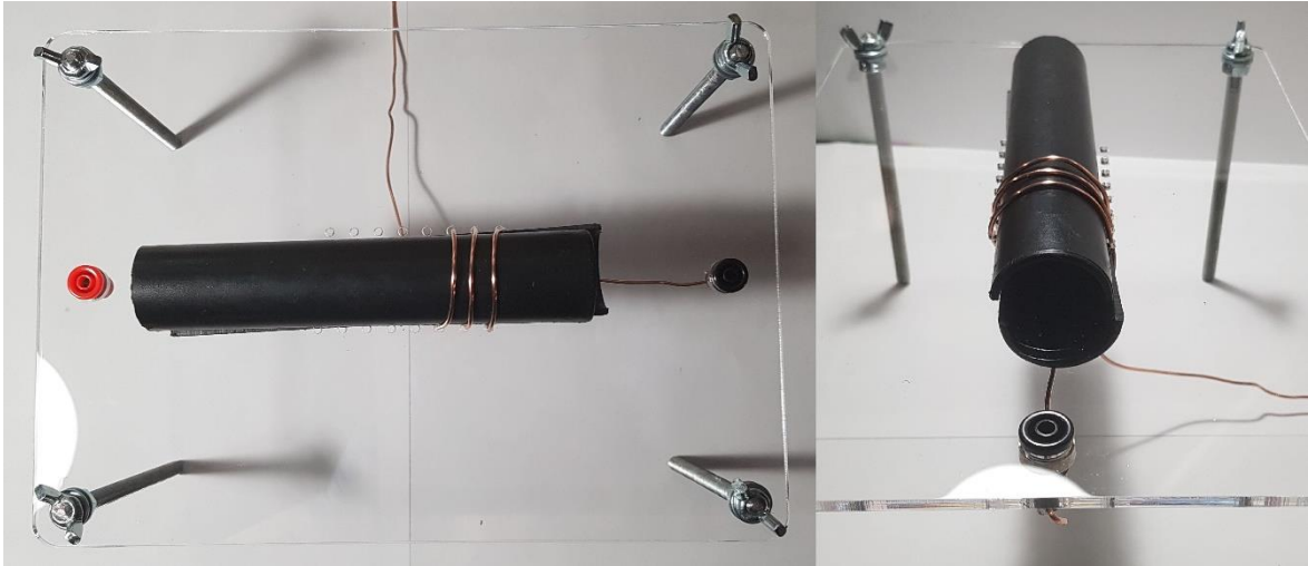
Slika 19 Namatanje zavojnice
