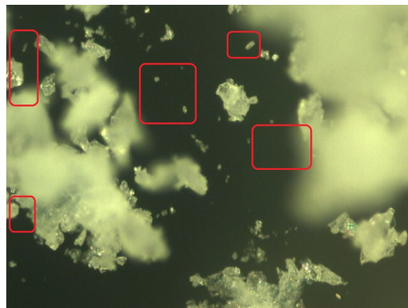
Slika 23. Dibromobenzene prije i nakon TO efekta
