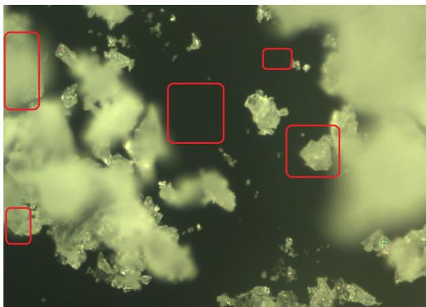
Slika 23. Dibromobenzene prije i nakon TO efekta
