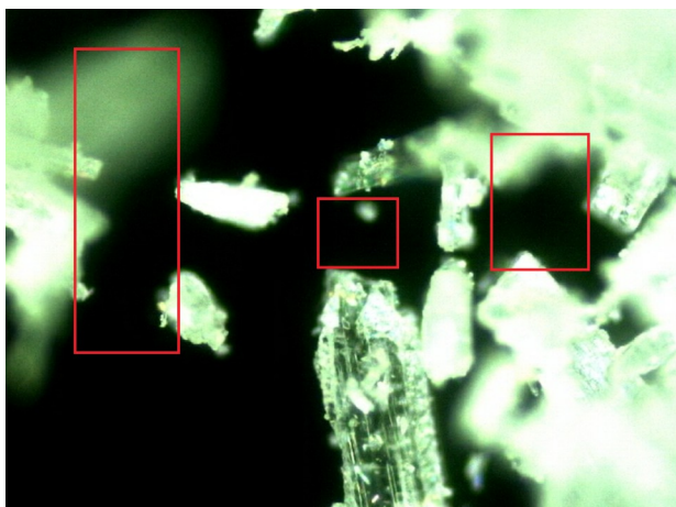
Slika 24. Tetraklorobenzen prije i nakon TO efekta
