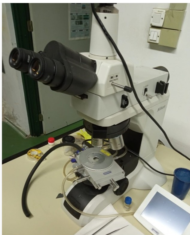
Slika 9. Mikroskop sa grijaćom pločom i komorom za hlađenje u laboratoriju za Mikrostrukturalna istraživanja na Prirodoslovno-matematičkom fakultetu u Zagrebu
