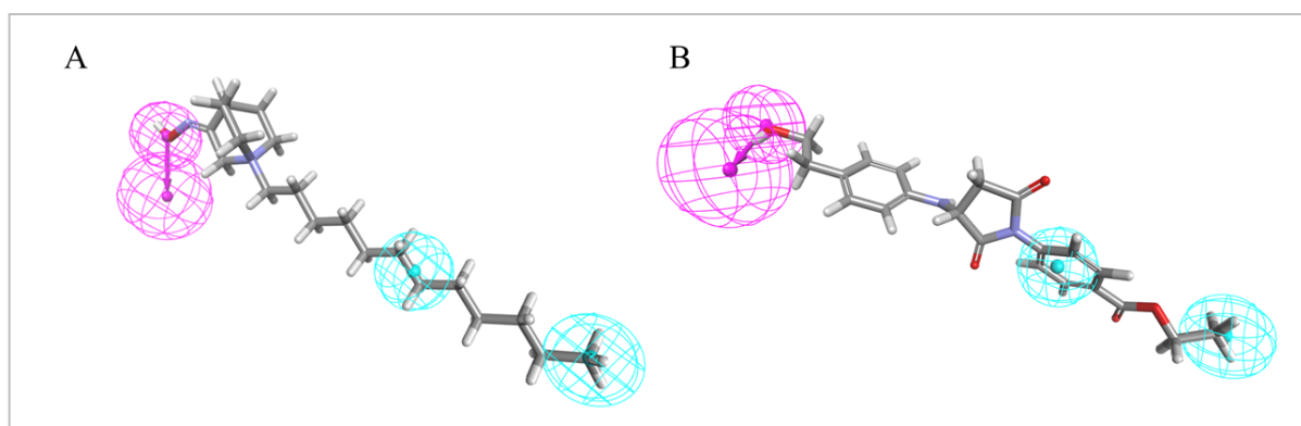
Slika 4.18. A) Kinuklidinijev oksim Q5 i B) Etil 4-(3-{[4-(2-hidroksietil)fenil]amino}-2,5-diokso-1-pirolidinil)benzoat mapirani na farmakoforni model za kinuklidinijevе oksime. Magenta označava donora vodikovih veza, a plavo hidrofobnu skupinu.
